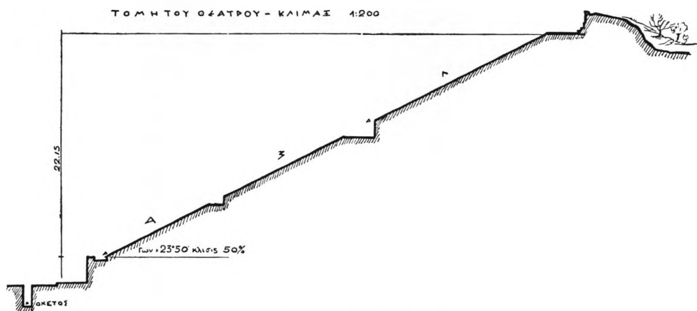
Σχέδ. 11. Τομή τοῦ κοίλου τοῦ θεάτρου
