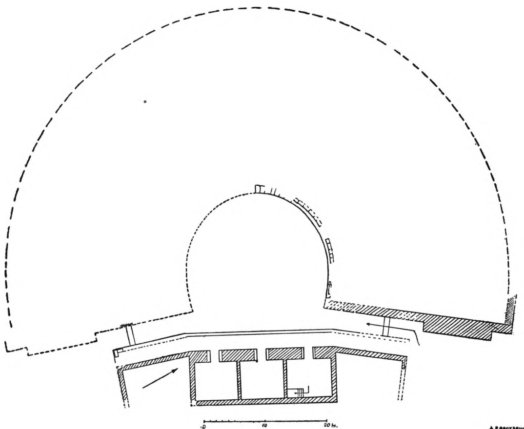
Σχ. 1. Δημητριάς. Κάτοψις τοῦ Θεάτρου (Ἀνασκαφαὶ 1958)
