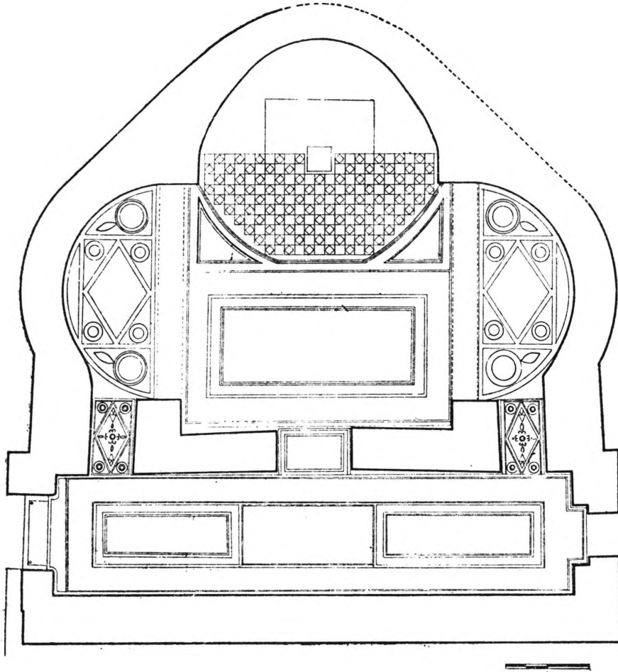
Τρίκογχος παλαιοχριστιανικός ναὸς Ἀκρινῆς. Κάτωψις
