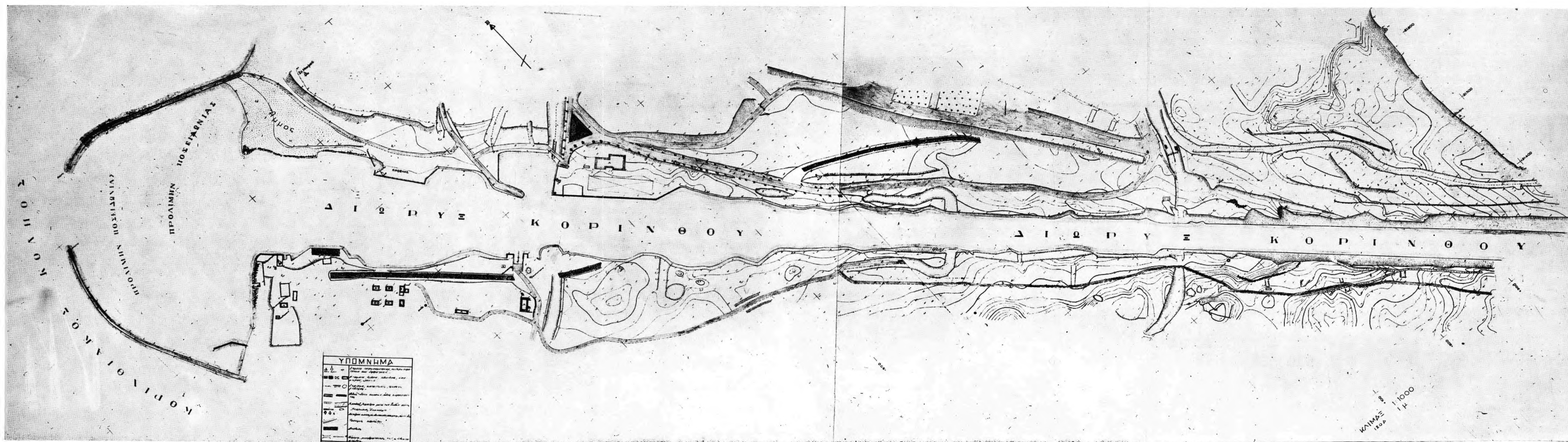
Σχεδιογράφημα Διώρυγος Κορίνθου καί τοῦ πέριξ αὐτῆς χώρου. Μὲ ἔντονον μελανὴν γραμμὴν σημειώνεται τὸ ἀποκαλυφθὲν τμήμα τοῦ Διόλκου
