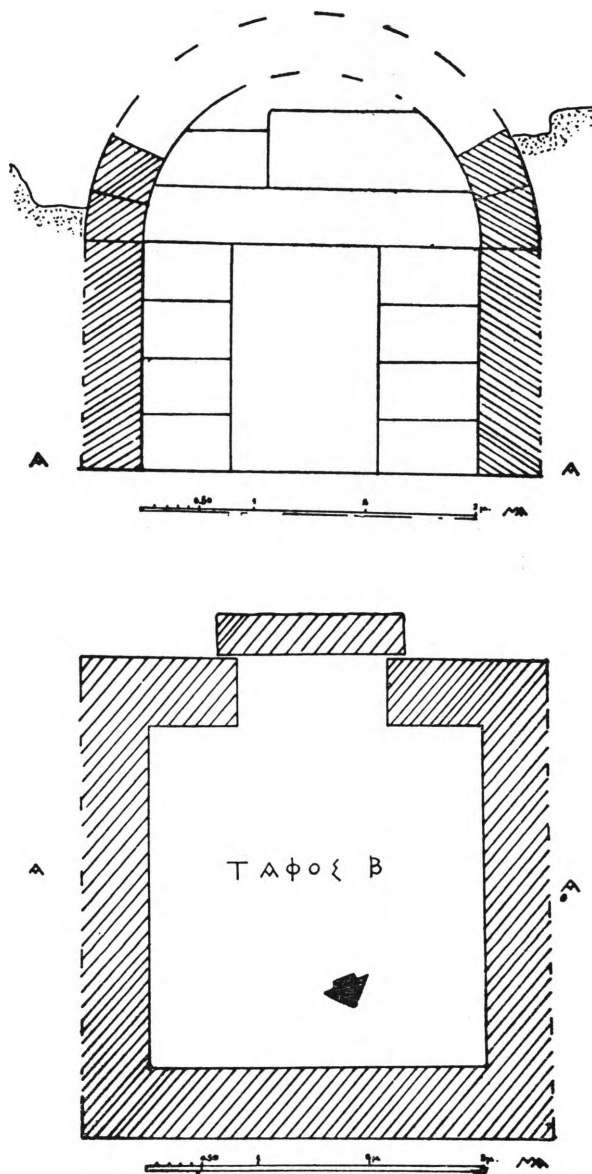
Σχ. 2. Τάφος Β Λακκώματος Χαλκιδικῆς
