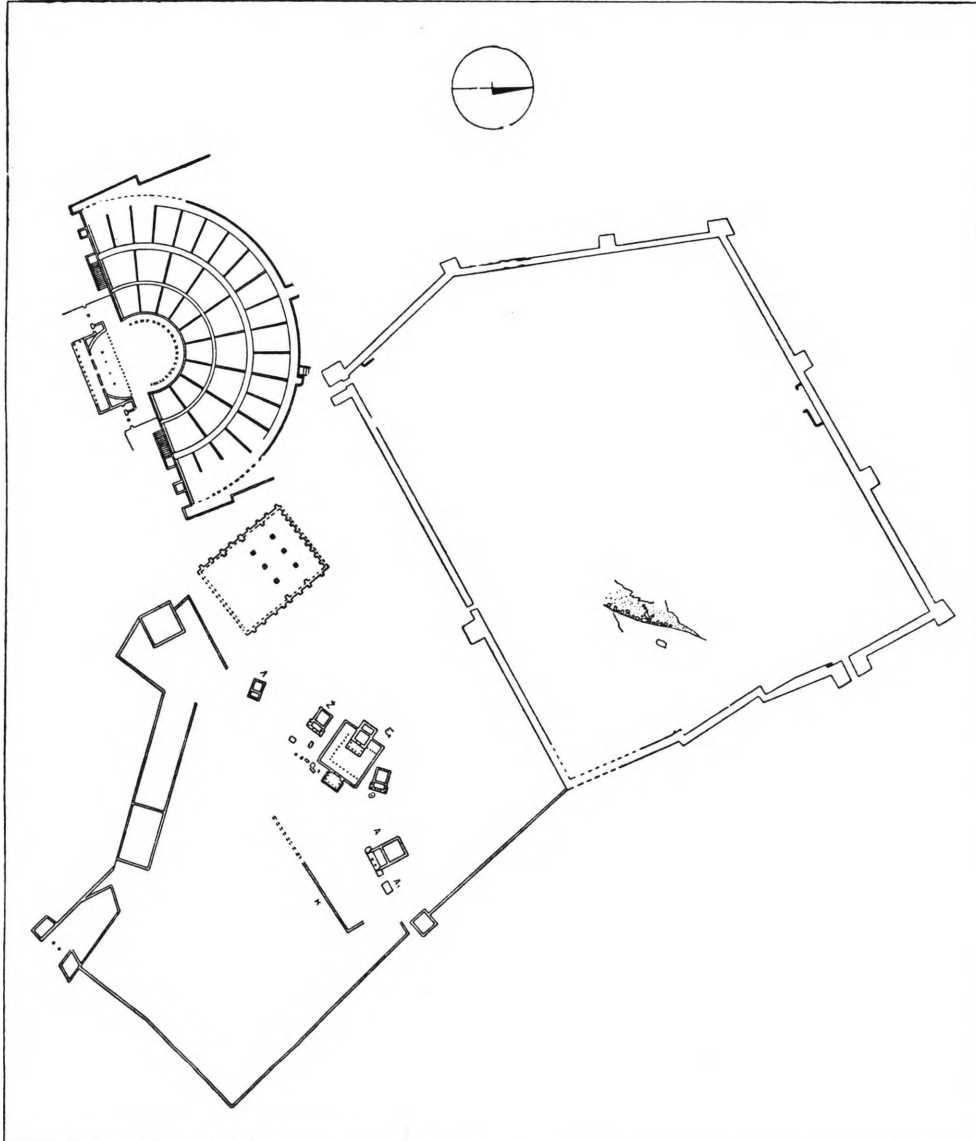
Σχέδ. 6. Κάτοπις τοῦ Ἱεροῦ περὶ τὸ τέλος τοῦ 3 ου π.Χ. αἰ.
