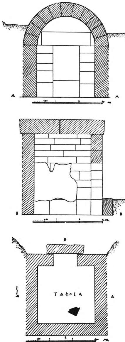
Σχεδ. 1. Τάφος Α Λακκώματος Χαλκιδικῆς. Κάτοψις καὶ τομαί
