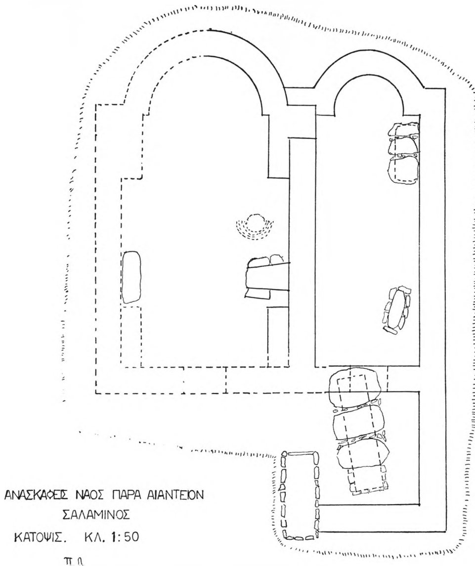
Σχεδ. 6. Ὁ παρά τὸ Αἰάντειον τῆς Σαλαμίνας ἀνασκαφεὶς ναὸς
