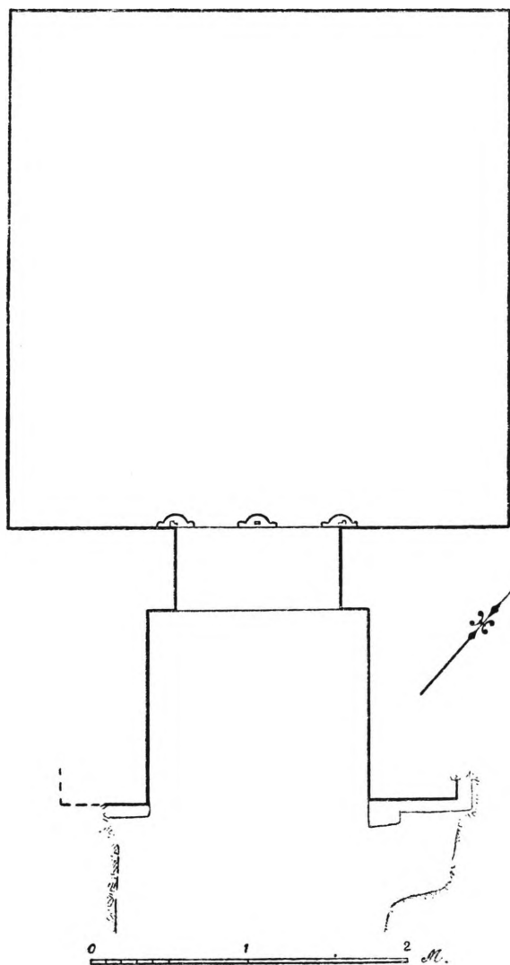
Σχ. 3. Κρανών. Κάτοψις τάφου Α
