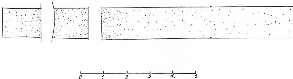
Σχεδ. Κρήνη Ἱεροῦ Ἀπόλλωνος ἐν Ζωστήρι
