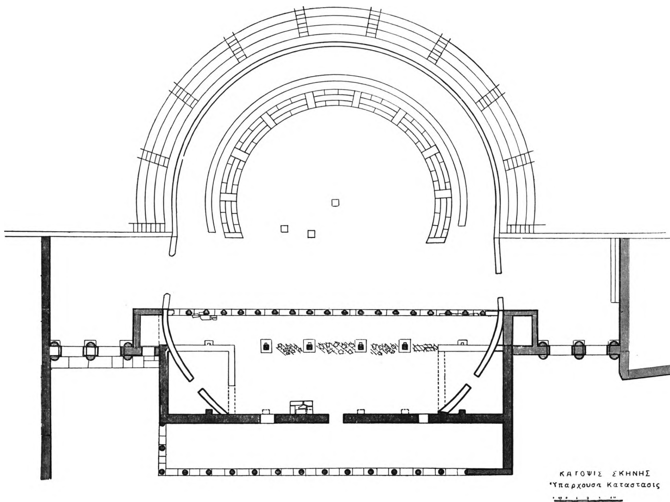
Σχέδ. 8. Κάτοπις θεάτρου (ὑπάρχουσα κατάσταση)
