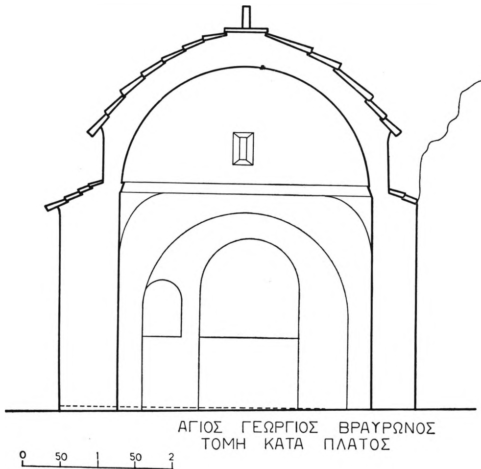
Σχεδ. 3. Κατὰ πλάτος τομὴ ναοῦ Ἁγίου Γεωργίου Βραυρῶνος
