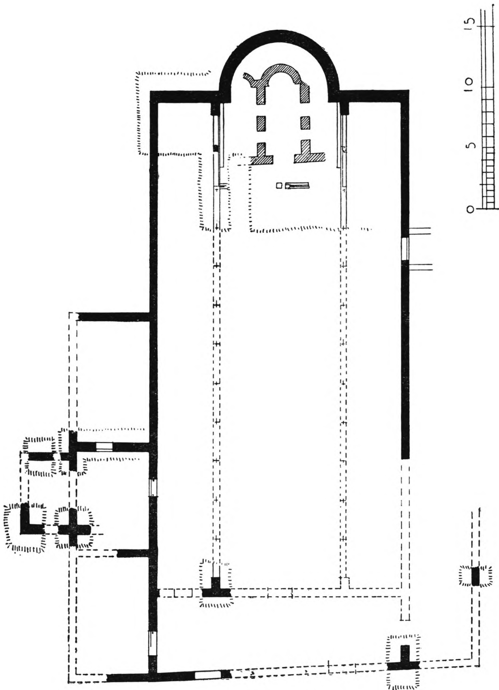
Σχεδιογράφημα Βασιλικής Ἀλίκας Ἀργους
