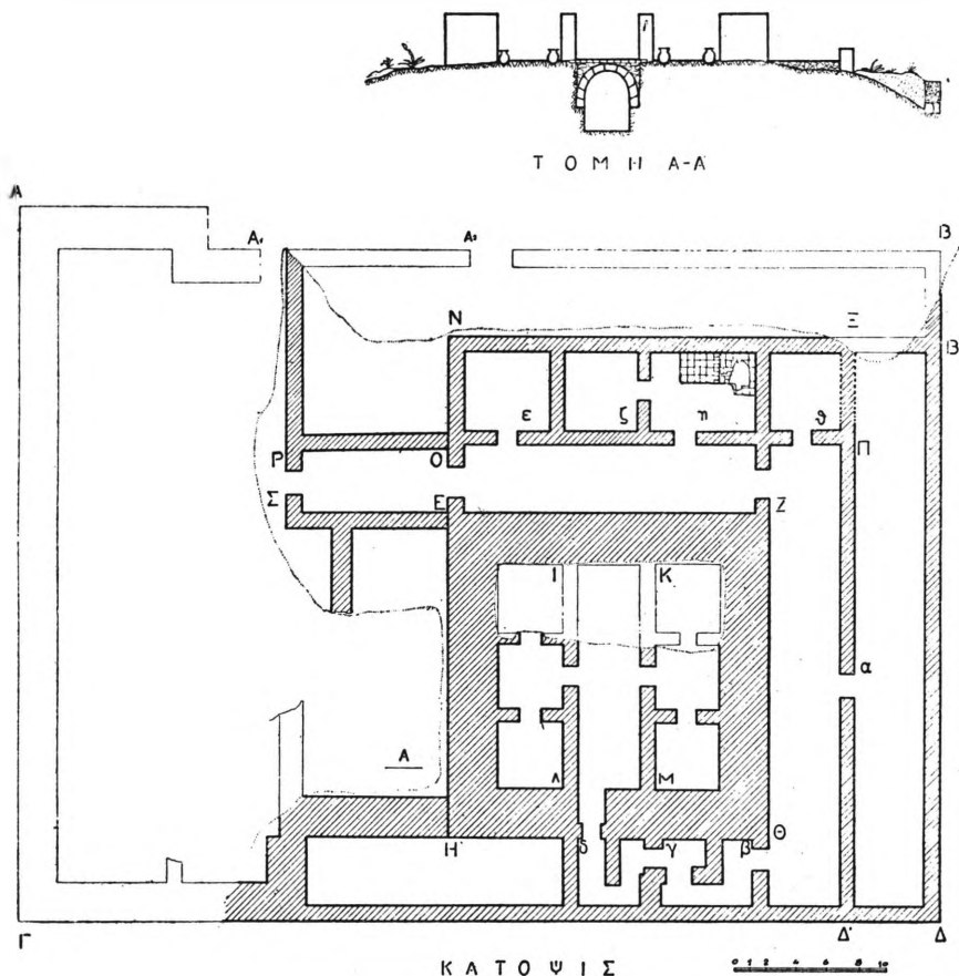
Σχ. 2. Κάτοψις Νεκυομαντείου Θεσπρωτικῆς Ἐφύρας
