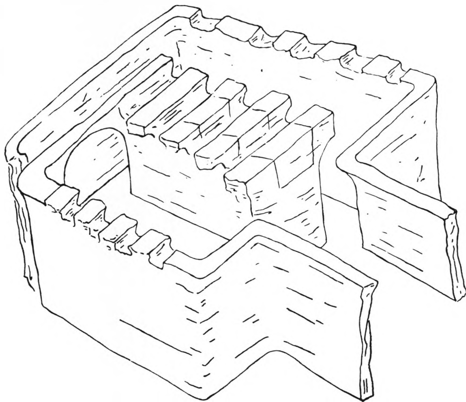
Σχέδ. 2. Προοπτικὸν σκαρίφημα τοῦ κεραμικοῦ κλιβάνου τοῦ Πίν. 50 β
