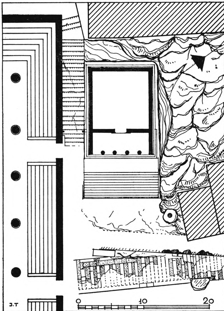
Σχεδ. 6. Ἀναπαραστάσις τοῦ θησαυροῦ τῆς Ἐλευσίνος
