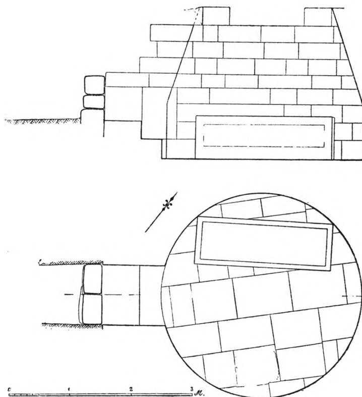
Σχ. 4. Κρανῶν. Τομή καὶ κάτοψις τάφου Β
