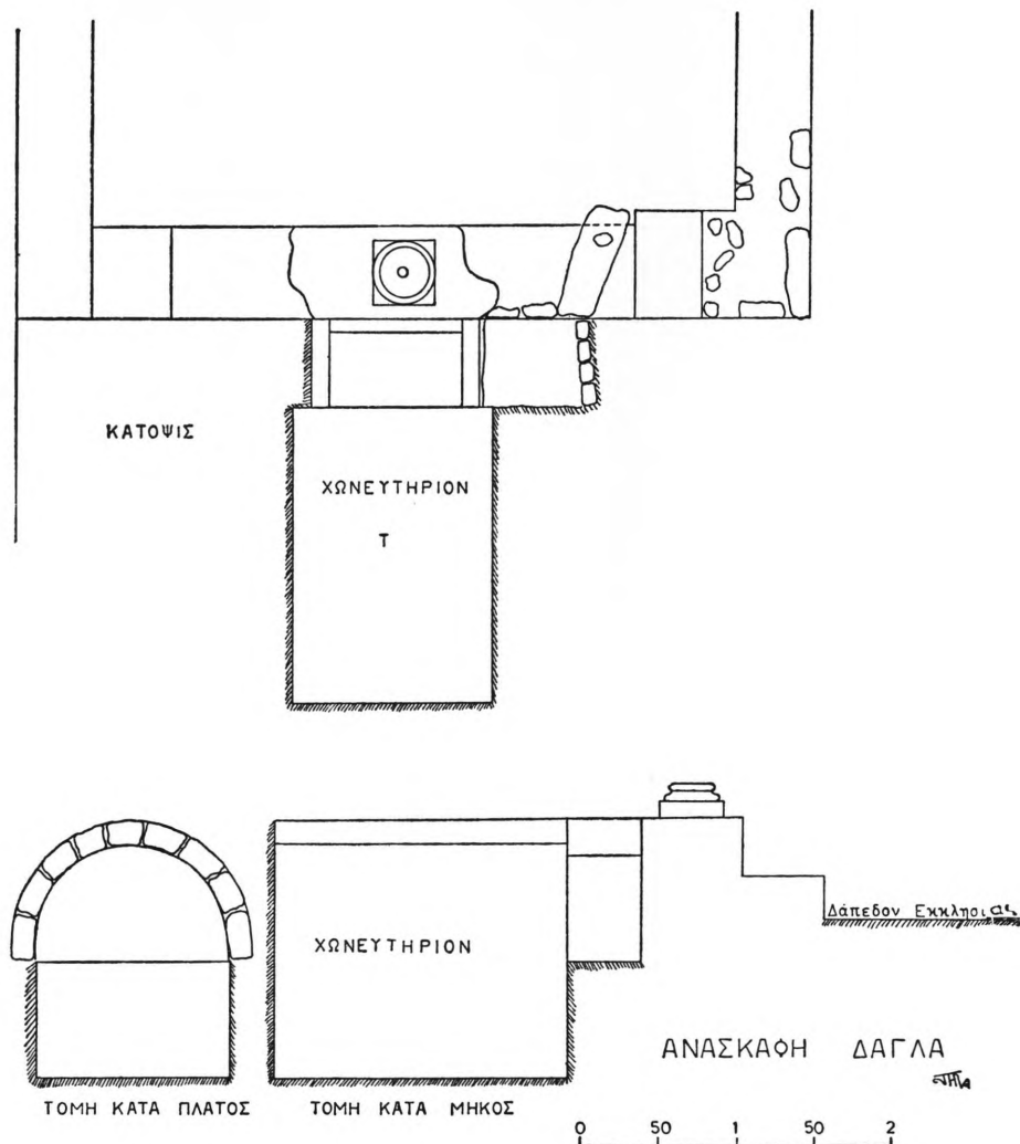
Σχεδ. 2. Κάτωψις καὶ τομαὶ κοινοῦ τάφου Ἁγίου Αἰμιλιανοῦ Δάγλα
