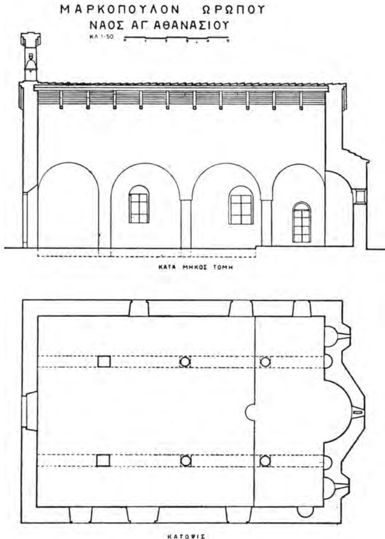
Σχέδ. 7. Μαρκόπουλον Ὁρωποῦ. Ναὸς Ἁγ. Ἀθανασίου. Τομὴ καὶ κάτοψις
