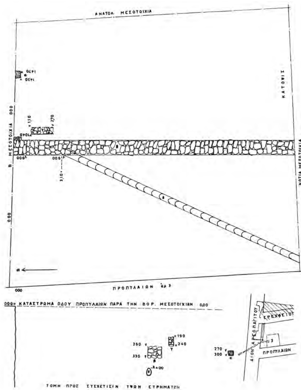
Σχέδ. 20. Άνασκαφή εν τῷ οἰκοπέδῳ Προπυλαίων 3 (Τομή 1 καὶ κάτωσις )
