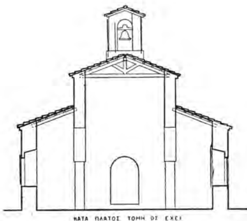
Σχέδ. 8. Μαρκόπουλον Ὠρωποῦ. Ναὸς Ἁγ. Ἀθανασίου. Δυτικὴ πρόσοψις καὶ τομαί
