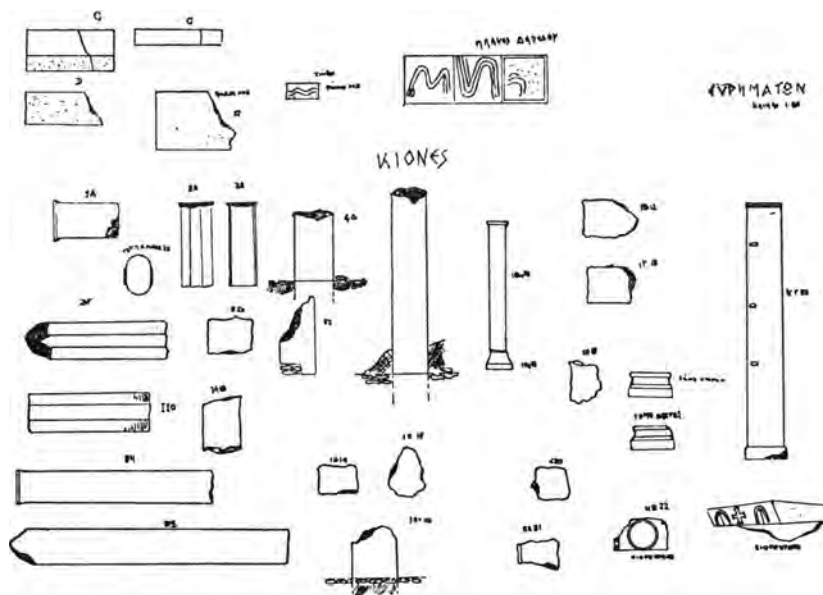
Σχέδ. 6. Σπάτα. Εὐρήματα ἀνασκαφείσης βασιλικῆς καὶ λεπτομέρειαι αὐτῶν
