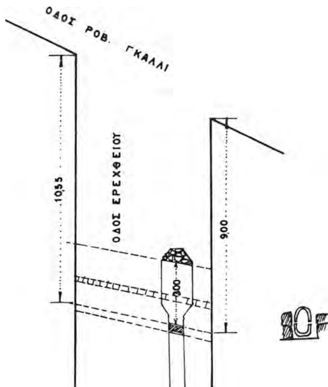
Σχέδ. 22. Κάτοψις καὶ τομὴ τοῦ ὑπὸ τὴν ὁδὸν Ἐρεχθείου πηλίνου ἀγωγοῦ
