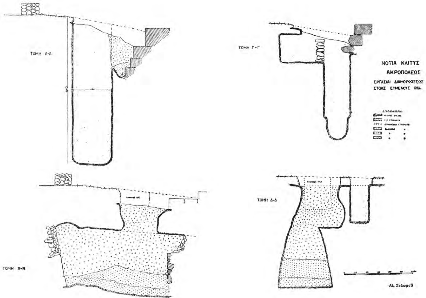
Σχέδ. 7. Τομαί τῆς ὑπ' ἀριθ. 6 κατόψεως
