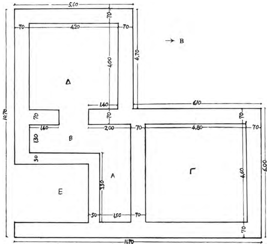
Σχέδ. 1. Κάτωρις Ρωμαϊκῆς ἐπαύλεως, ἀποκαλυφθείσης εἰς οἰκόπεδον Παρασκευοπούλου εἰς Σπάρτην
