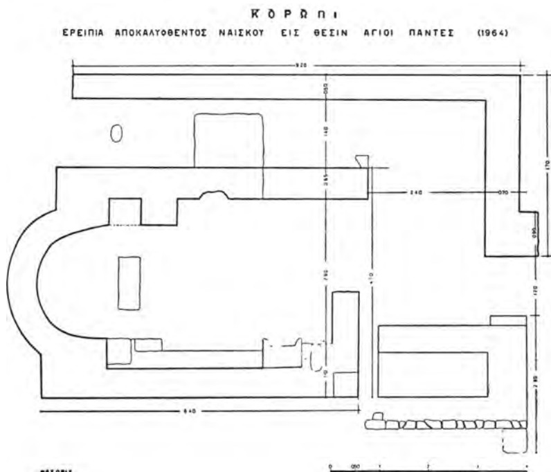
Σχέδ. 4. Κορωπί. Ἐρείπια ναῖσκου εἰς θέσιν Ἁγιοὶ Πάντες
