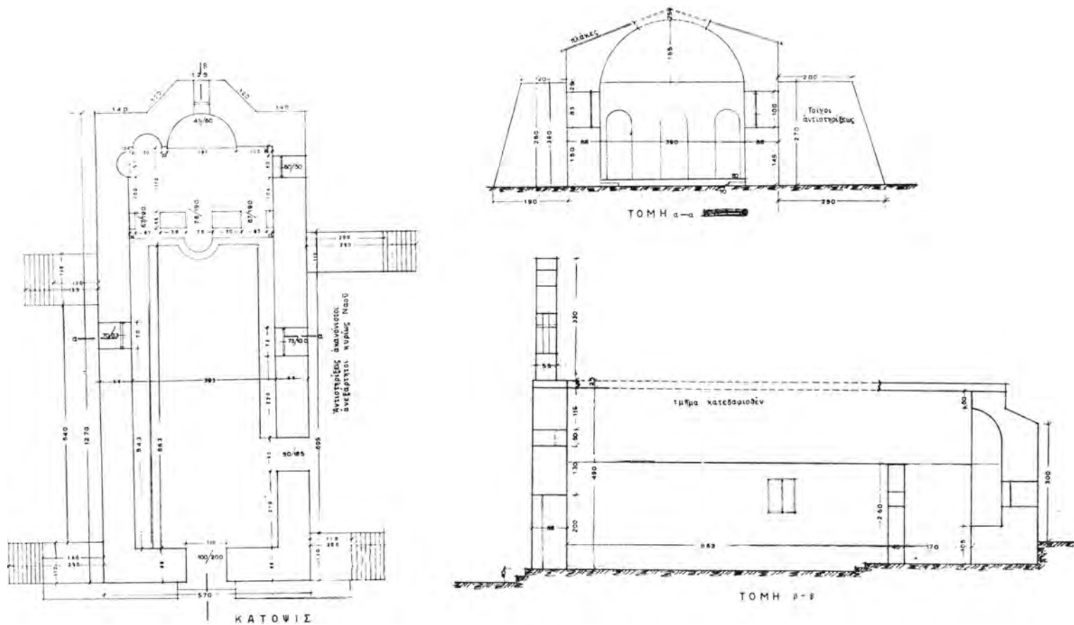
Σχέδ. 1. Κάτωψις καὶ τομαὶ ναοῦ Ἁγίου Ἰωάννου τῶν Μαυρομιχαλαίων ἐν Ἀρεσπόλει Λακωνίας
