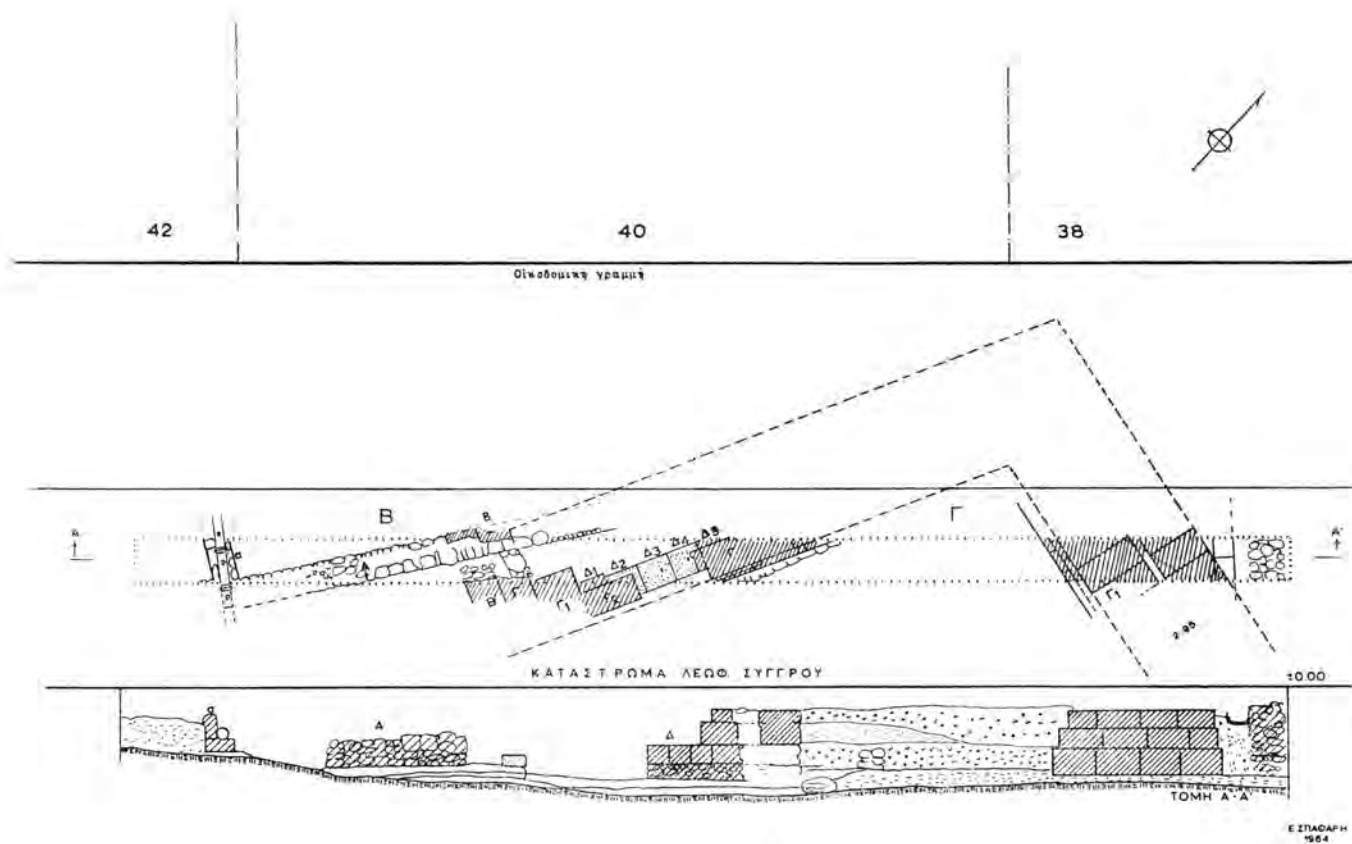
Σχέδ. 30. Κάτοψις και τομή αρχαίου τείχους
