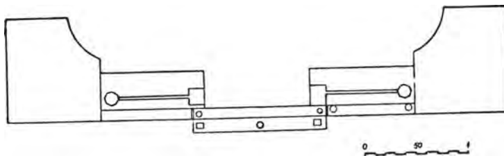
Σχέδ. 2. Μονὴ Νταοῦ Πεντέλης. Κάτωψις κρηπιδώματος τέμπλου
