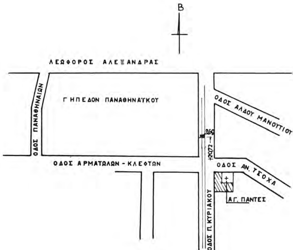
Σχέδ. 35. Τοπογραφικὸν διάγραμμα τοῦ χάνδακος τῆς ΥΔΡΕΞ, ὅπου εὗρέθησαν τὰ χάλκινα ἀγαλμάτια
