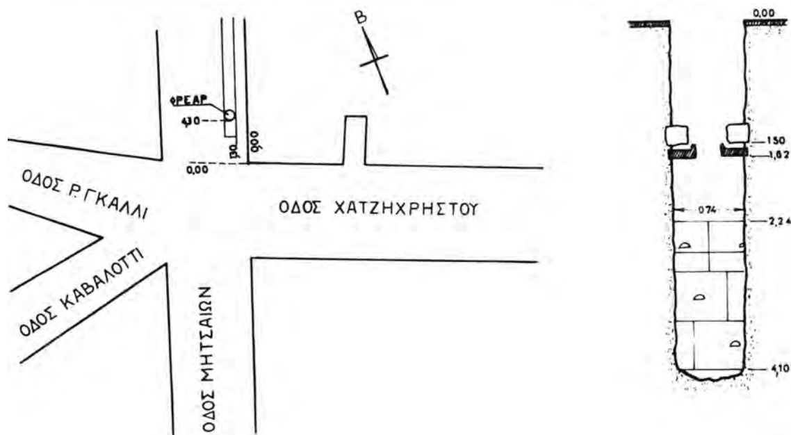
Σχέδ. 19. Θέσις εὐρέσεως ἀρχαίου φρέατος καὶ τομὴ αὐτοῦ
