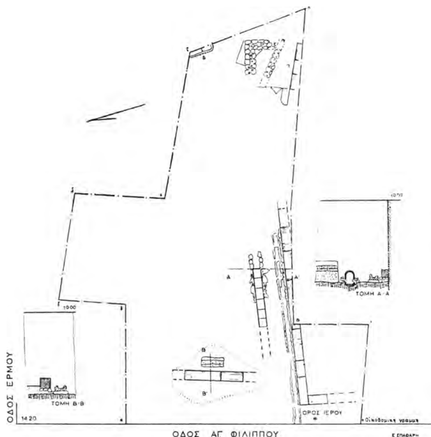
Σχέδ. 7. Κάτοπις ἀνασκαφῶν ἐν οἰκοπέδῳ τῆς ὁδοῦ Ἀγ. Φιλίππου
