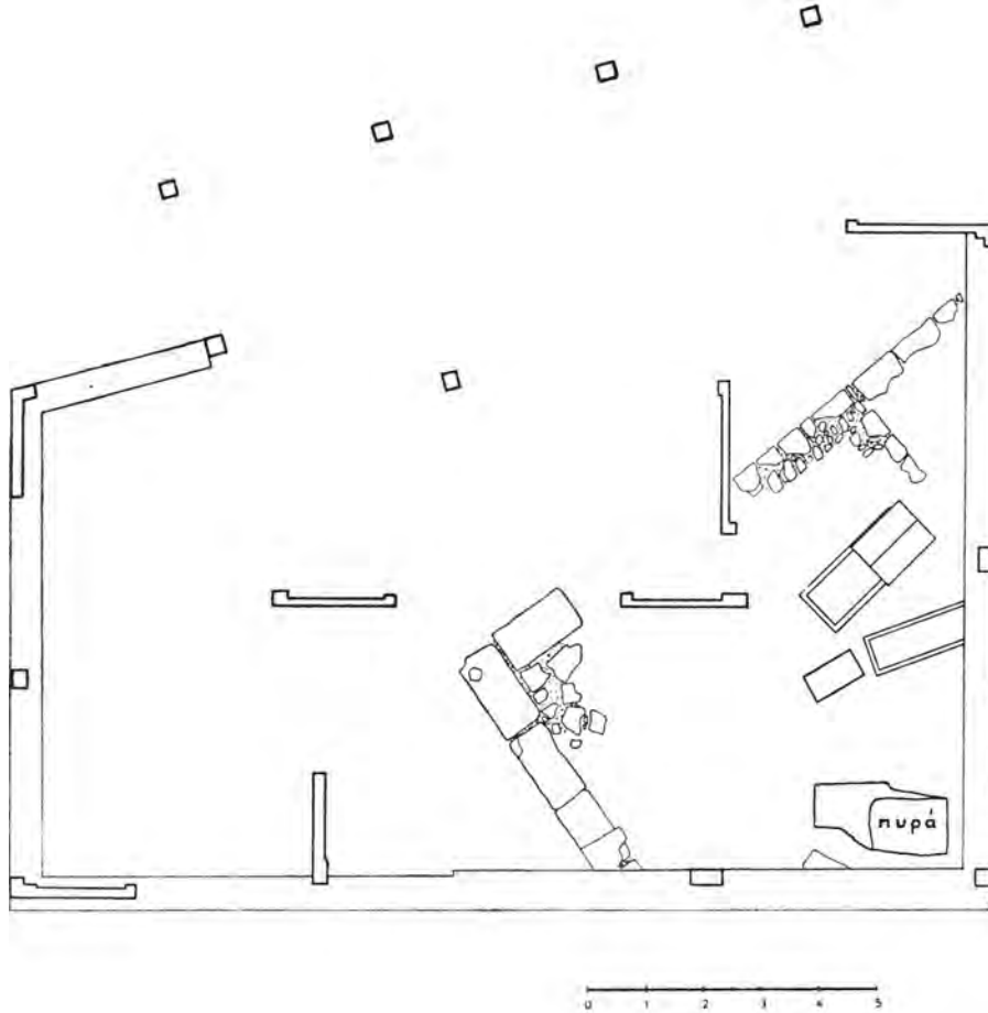
Σχέδ. 1. Κάτοψις τάφων Βούλας
