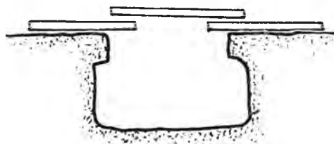
Σχέδ. 14. Τομὴ ἀγωγοῦ Ἀδριανείου ὕδραγωγείου
