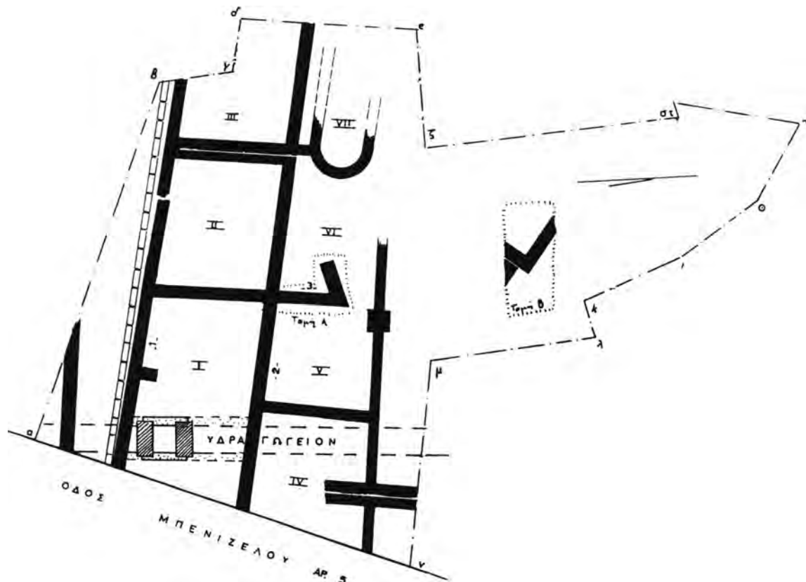
Σχέδ. 13. Κάτοψις τοῦ παρὰ τὴν ὁδὸν Μπενιζέλου ὑστερορρωμαϊκῶν χρόνων κτηρίου
