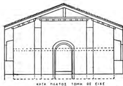
Σχέδ. 8. Μαρκόπουλον Ὠρωποῦ. Ναὸς Ἁγ. Ἀθανασίου. Δυτικὴ πρόσοψις καὶ τομαί
