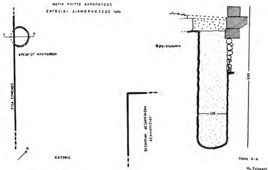
Σχέδ. 5. Κάτωψις καὶ τομή τοῦ Β. τῆς Στοᾶς Εὐμένους μυκηναϊκοῦ φρέατος ΣΤ'
