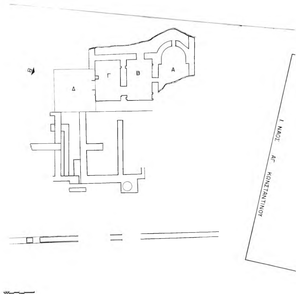
Σχέδ. 1. Ἅγιος Κωνσταντῖνος Λοκρίδος. Κάτοψις ἐρειπίων λουτρῶνος
