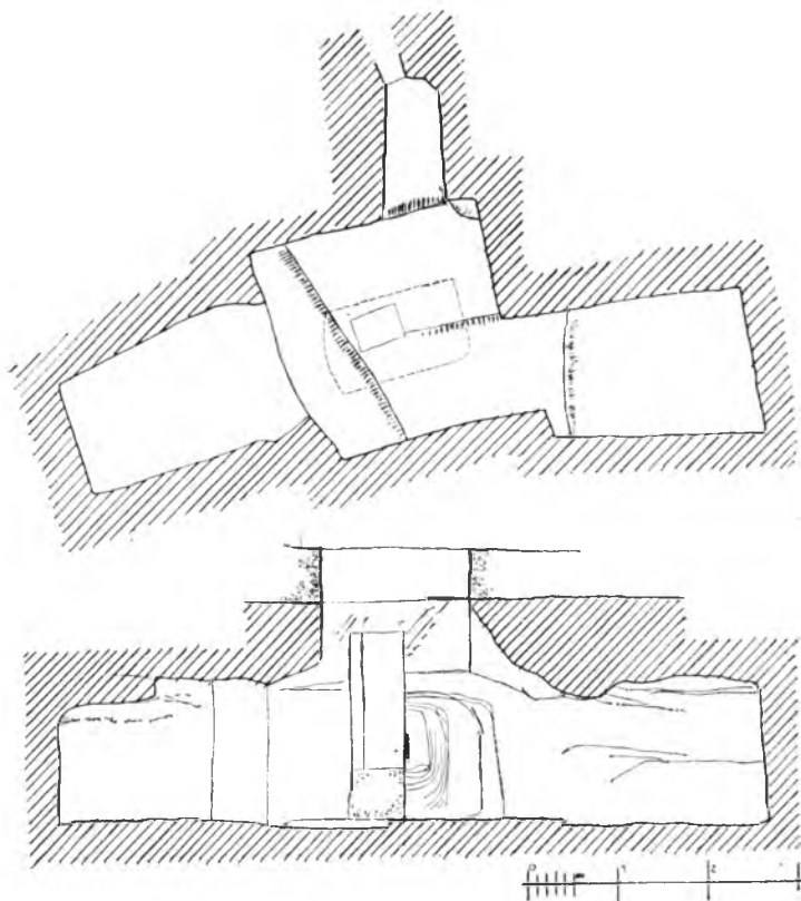
Σχέδ. 3. Αίγινα, θέσις Μύλοι. Κάτοψις καὶ τομή τάφου 2
