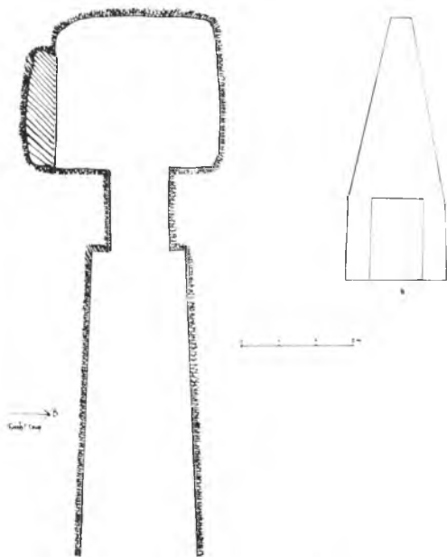
Σχέδ. 4. Θῆβαι. Κάτοπις καὶ ὄπισ θάλαμοι- δοὺς μυκηναϊκοῦ τάφου ἀποκαλυφθέντος εἰς τὸν λόφον τοῦ Μεγάλου Καστελλίου (Γηροκομεῖον)
