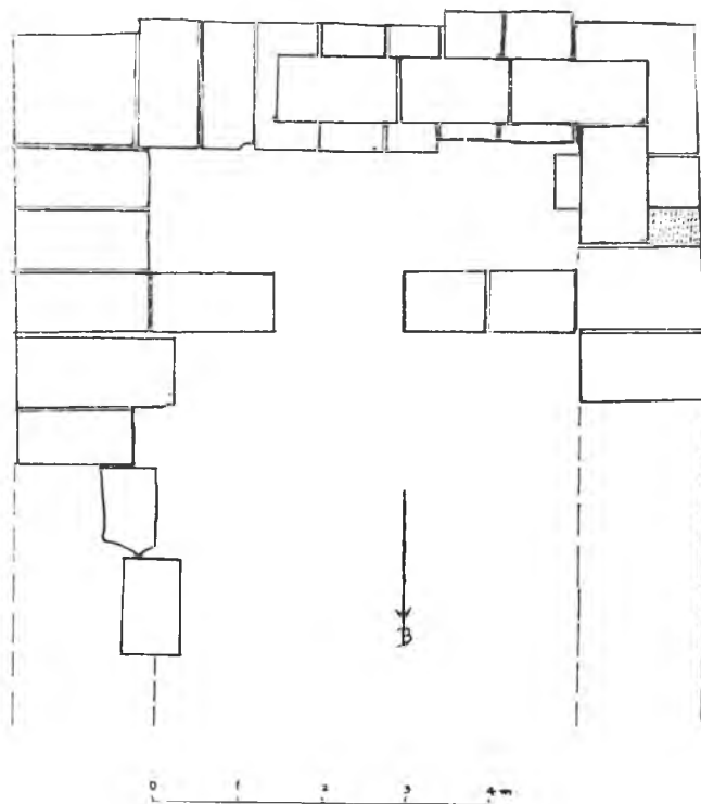
Σχέδ. 11. Λαμία, οἰκόπ. Χ. Κοκκαλάκη. Κάτοψις ναῖσκου
