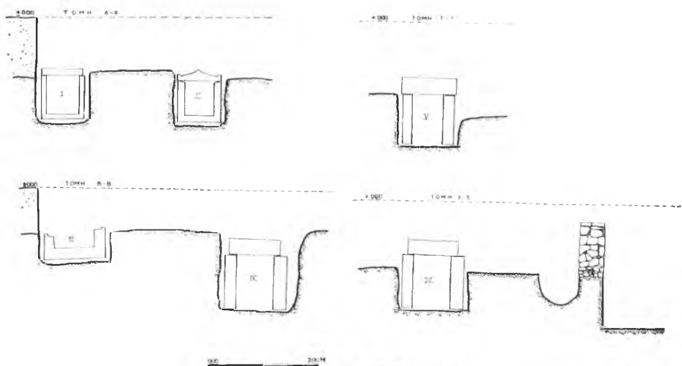
Σχέδ. 30. Τομαὶ τάφων, ἀποκαλυφθέντων ἐπὶ τῆς ὁδοῦ Μυλλέρου 16 - 18 (πρβλ. Σχέδ. 28)
