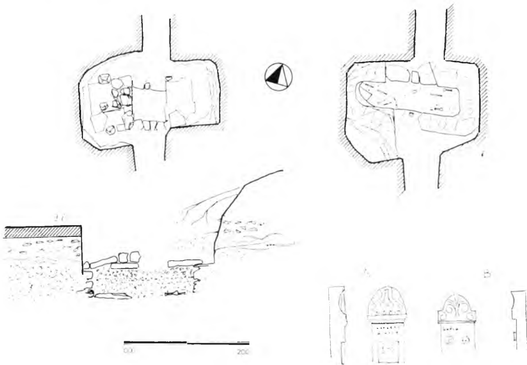
Σχέδ. 3. Ἐλευσίς. Ὁδὸς Θηβῶν 611. Κατόψεις καὶ τομὴ τάφου, ὡς καὶ ὄψιν καὶ πλαγία τομὴ ἐπιτυμβίων στηλῶν - καλυμμάτων τούτου
