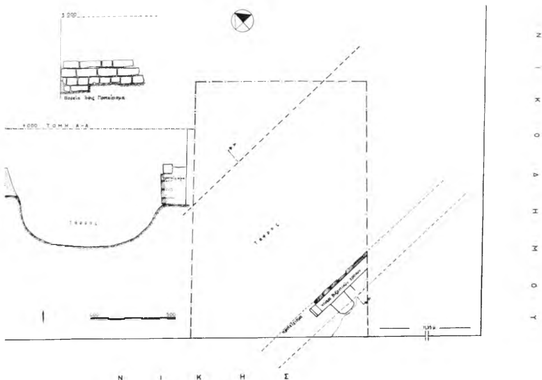
Σχέδ. 32. Κάτοψις, τομή καὶ ὄψις τμήματος τοῦ προτειχίσματος καὶ τῆς πρὸ αὐτοῦ τάφρου ἐπὶ τῆς ὁδοῦ Νίκης 27
