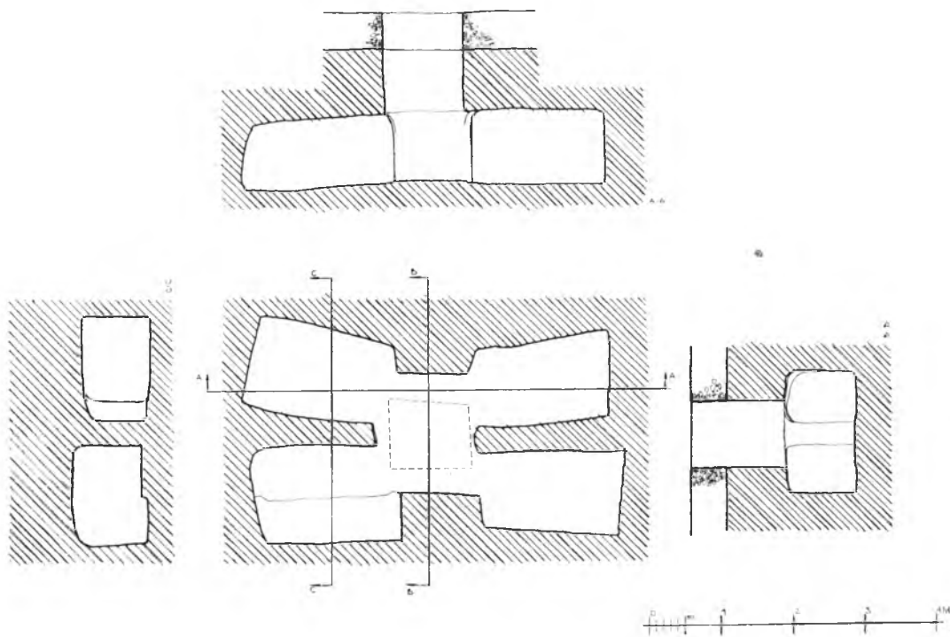
Σχέδ. 2. Αἶγινα, θέσις Μύλοι. Κάτωψις καὶ τομαὶ τάφου 1
