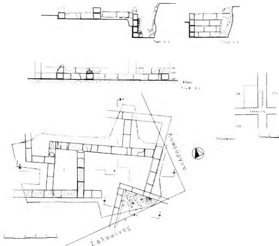
Σχέδ. 11. Μέγαρα. Ὁδὸς Σαλαμίνιος καὶ Λυκούργου. Κάτοψις, τομαὶ καὶ τοπογραφικὸν σχεδιογράφημα ἀνασκαφῆς
