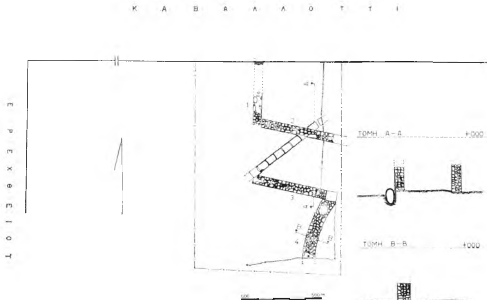
Σχέδ. 22. Κάτοψις καὶ τομαὶ τοίχων, ἀποκαλυφθέντων εἰς οἰκόπεδον ἐπὶ τῆς ὁδοῦ Καβαλλόττι 9
