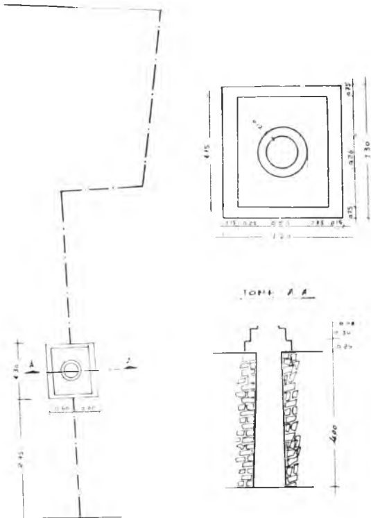
Σχέδ. 12. Λαμία. Κάτωψις καὶ τομὴ κτιστοῦ φρέατος ἀποκαλυφθέντος ἐν οἰκοπέδῳ Φουρλιᾶ
