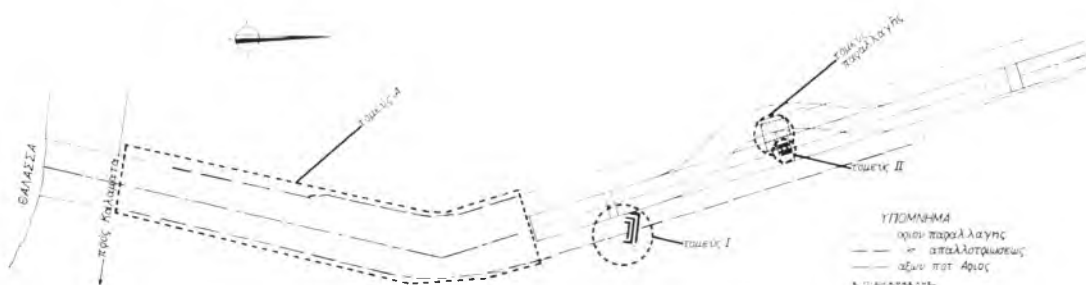
Σχέδ. 1. Ἀκοβίτικα Μεσσηνίας. Τοπογραφικὸν διάγραμμα τῆς κοίτης - διώρυγος τοῦ ποταμοῦ Ἄριος
