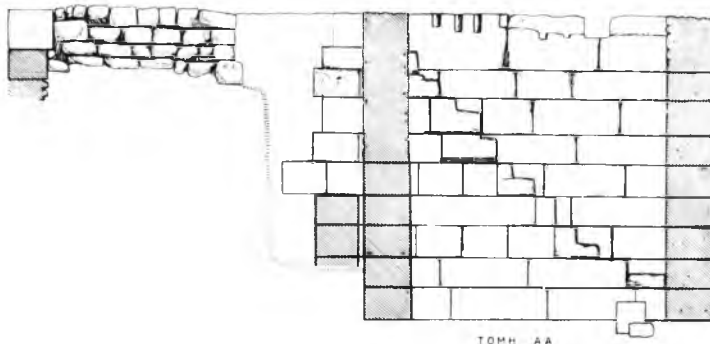
Σχέδ. 13. Μέγαρα. Ὁδὸς Μινώας 23. Τοπογραφικὸν σχεδιογράφημα καὶ τομὴ ἐλληνιστικοῦ οἰκοδομήματος (πρβλ. Σχέδ. 12)
