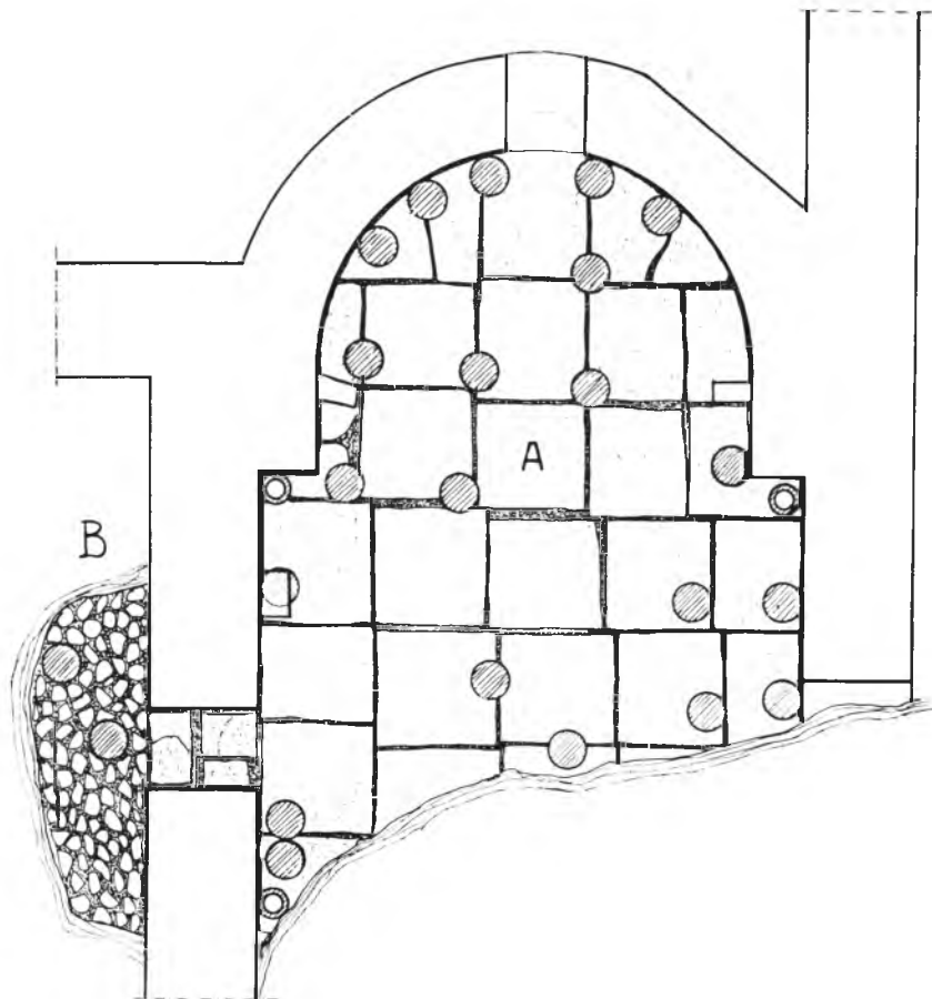
Σχέδ. 2. Ἁγιος Κωνσταντῖνος Λοκρίδος. Κάτοπις ὑποκαύστου λουτρῶνος
