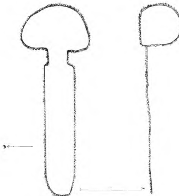
Σχέδ. 13. Ἀγναντῆ Λοκρίδος. Κάτωψις καὶ τομὴ θαλαμοειδοῦς μυκηναϊκοῦ τάφου
