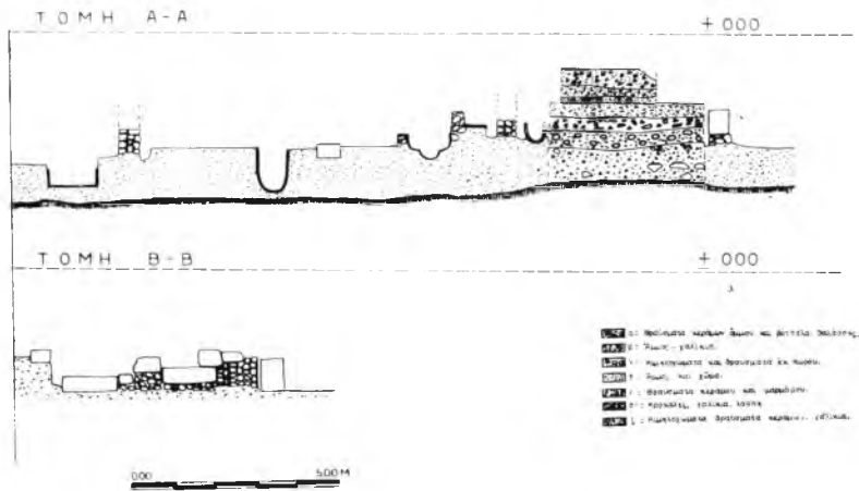
Σχέδ. 20. Τομαί ανασκαφής επί της οδού 'Ηρακλειδών 15-17 (πρβλ. Σχ έδ. 19)
