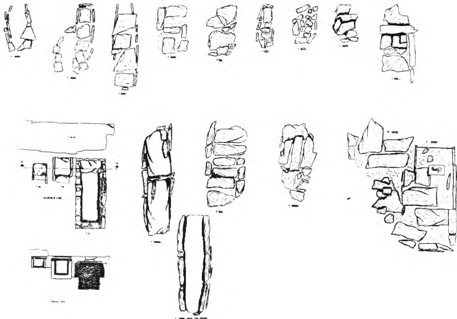
Σχέδ. 6. Ἀνάβυσσος. Σχεδιαστική ἀποτύπωσις τῶν τύφων XXIII, XXV, XIV, XVII, XL, XLI, XLII, XLIV, XIII, III, II, I, XXIX, XV, XXVI, XXXII, XXXI
