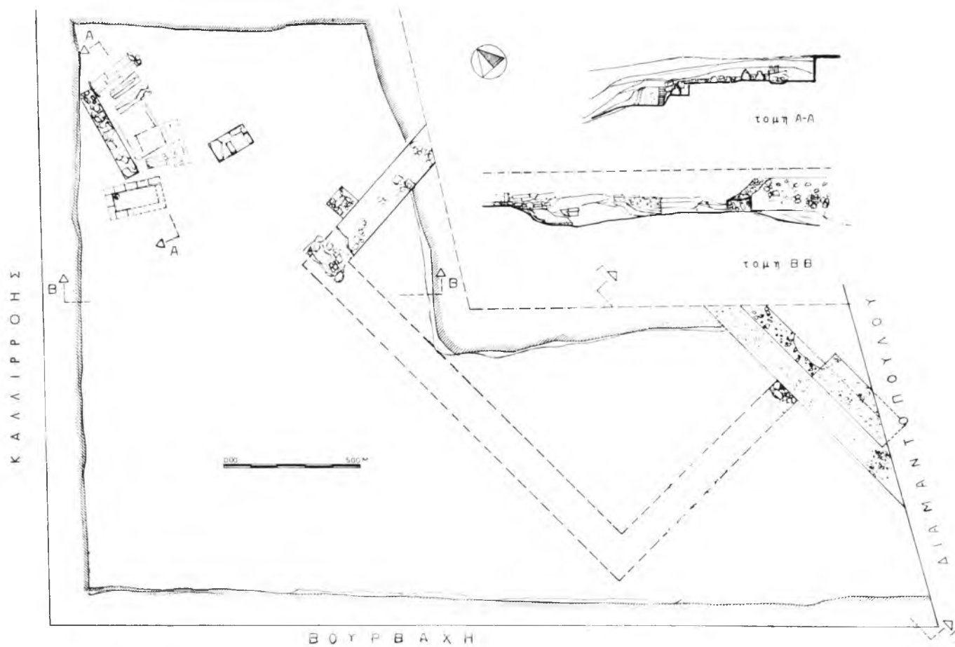
Σχέδ. 12. Κάτοψις και τομαί του Γυμνασίου του Κυνოსάργους, ἀποκαλυφθέντος ἐπὶ τῶν ὁδῶν Βούρβαχη - Καλλιρρόης - Διαμαντοπούλου
