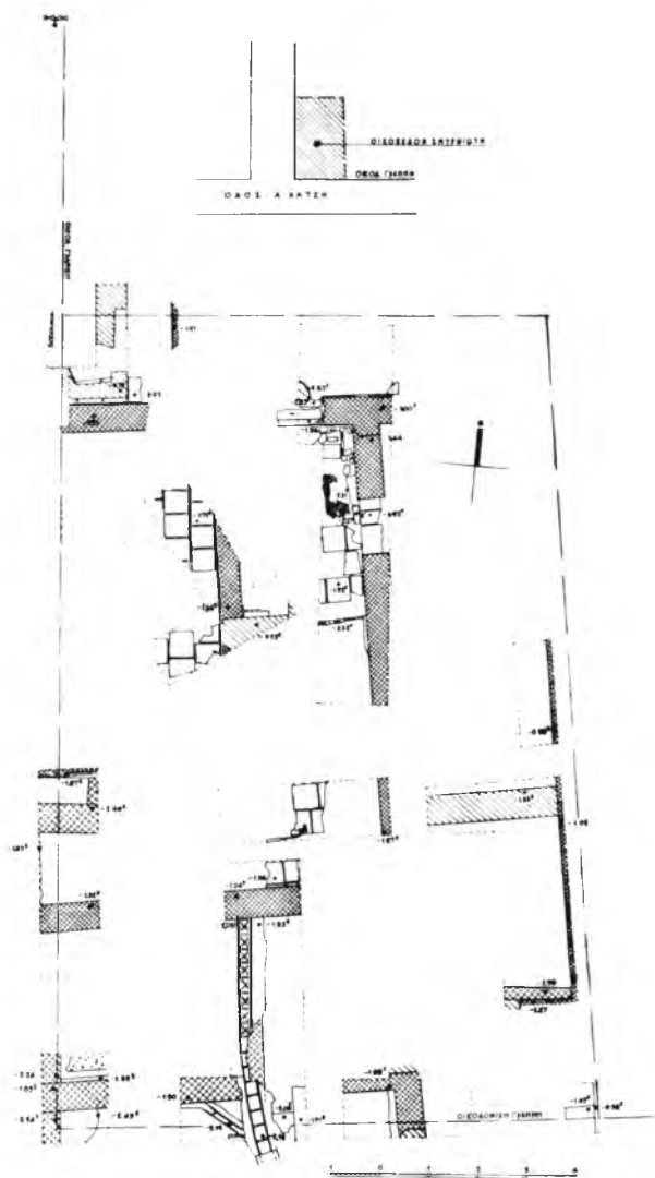
Σχέδ. 1. Ἄργος. Τοπογραφικὸν διάγραμμα καὶ κάτοψις ἀνασκαφῆς εἰς οἰκόπεδον Σμυρνιώτη
