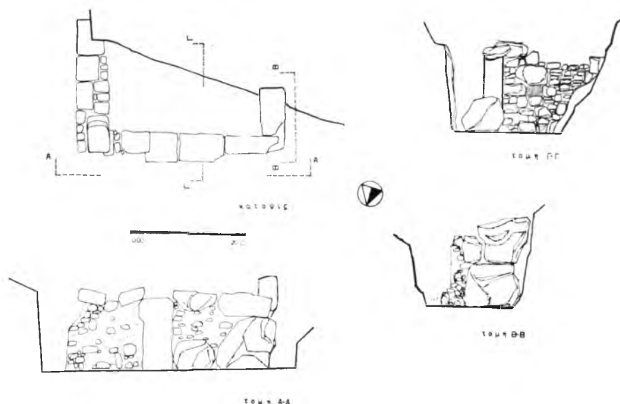
Σχ. ἐδ. 9. Μέγαρο. Κάτοψις καὶ τομαὶ ἀνασκαφῆς ἐπὶ τῆς ὁδοῦ Δογάνη 30
