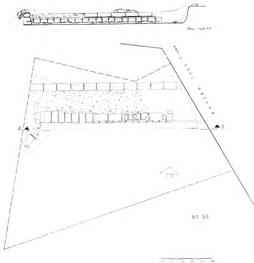
Σχέδ. 7. Μέγαρο (Ο.Τ. 56). Κάτωψις και τομή τμήματος του αρχαίου τείχους της πόλεως
