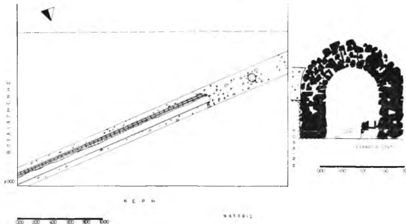
Σχέδ. 31. Κάτοψις καὶ τομή τμήματος ὑστερορρωμαϊκοῦ ὑδραγωγείου, ἀποκαλυφθέντος ἐπὶ τῶν ὁδῶν Νέρη 11 καὶ Βουλιαγμένης
