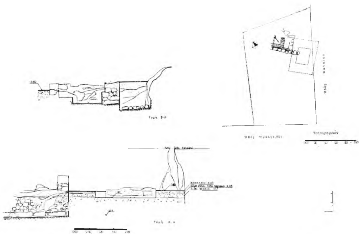
Σχέδ. 18. Τοπογραφικὸν διάγραμμα περιοχῆς καὶ τομαὶ κτισμάτων, ἀποκαλυφθέντων ἐπὶ τῶν ὁδῶν Ἡρακλειδῶν καὶ Ἀκταίου (πρβλ. Σχέδ. 17)
