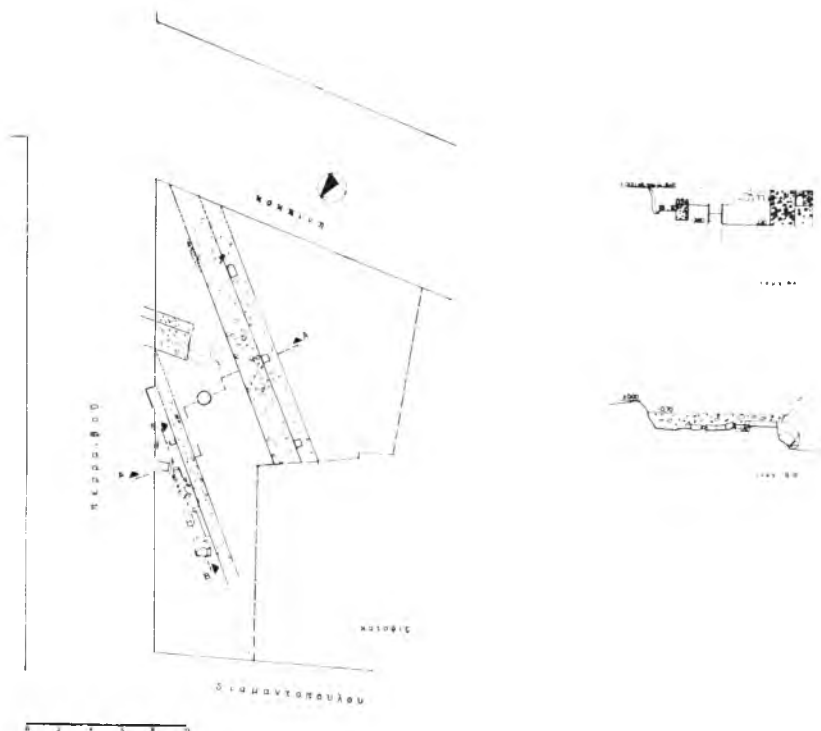
Σχέδ. 23. Κάτωψις καὶ τομαὶ τμήματος τοῦ Γυμνασίου τοῦ Κυνοςάργου ἐπὶ τῶν οδῶν Κοκκίνη - Περραιβοῦ - Διαμαντοπούλου
