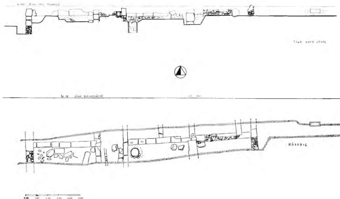
Σχέδ. 14. Μέγαρο. Ὁδὸς Μυκηνῶν. Κάτοψις καὶ τομὴ ἀρχιτεκτονικῶν λειψάνων καὶ τμήματος ἀρχαίας ὁδοῦ
