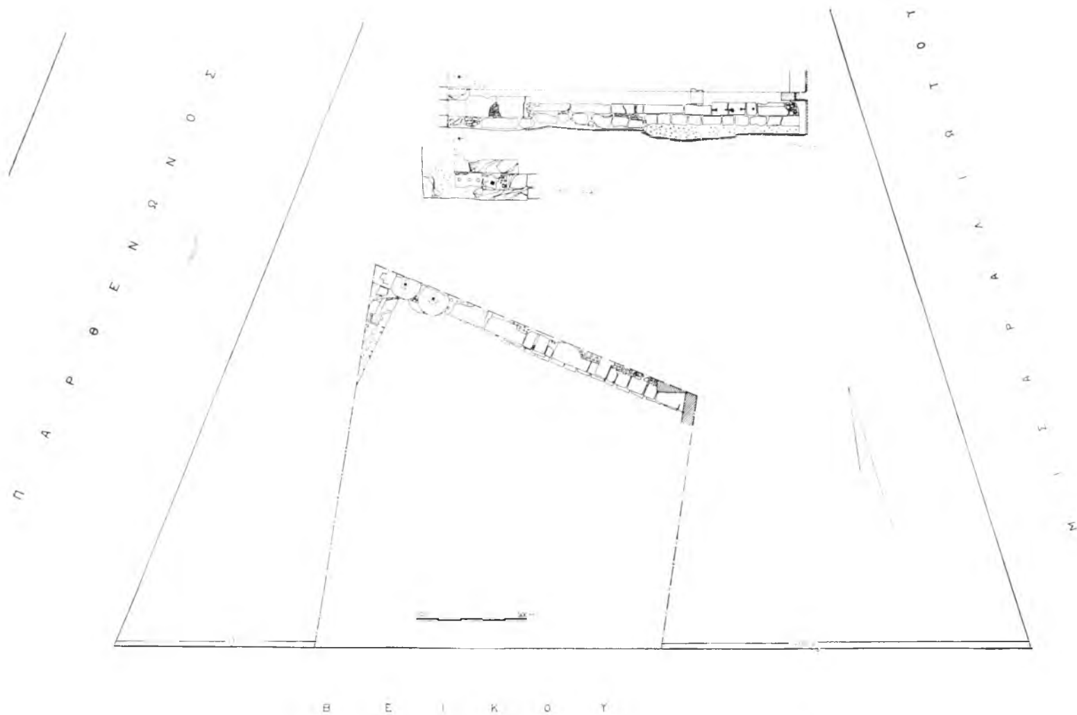
Σχέδ. 4. Κάτοψις, κυρία ὄψις καὶ τομή τμήματος τοῦ τείχους τῆς πόλεως, ἀποκαλυφθέντος ἐπὶ τῆς ὁδοῦ Βεΐκου 24-26
