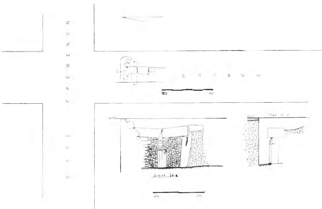
Σχέδ. 10. Μέγαρο. Ὁδὸς Δογάνη. Κάτωφλις, δυτικὴ ὄψις καὶ τομὴ ἐλληνιστικοῦ ὑπογείου κτίσματος
