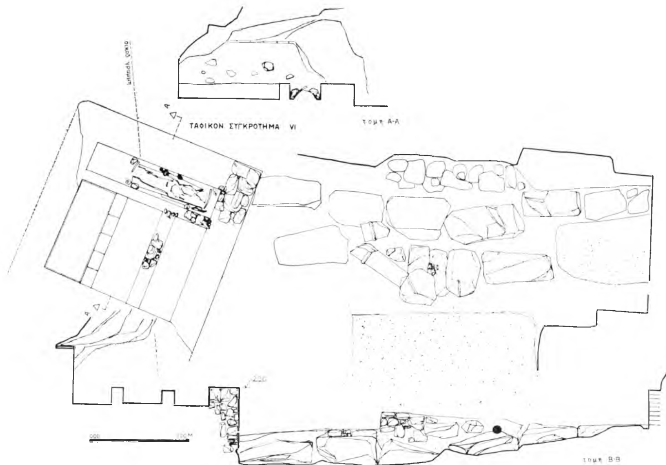
Σχέδ. 10. Κάτοψις και τομαί ταφικοῦ συγκροτήματος VI, ἀποκαλυφθέντος ἐπὶ τῶν ὁδῶν Βούρβαχη 24-26 καὶ Κοκκίνη
