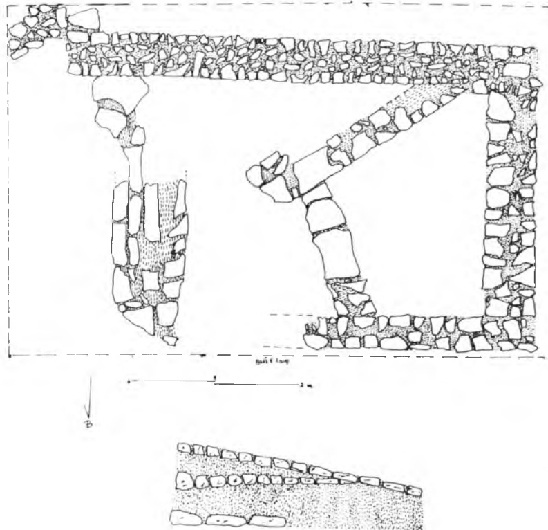
Σχέδ. 1. Θῆβαι, οἰκόπ. Δαγδελῆνη. Κάτοψις καὶ τομὴ τοίχων μυκηναϊκῶν χρόνων
