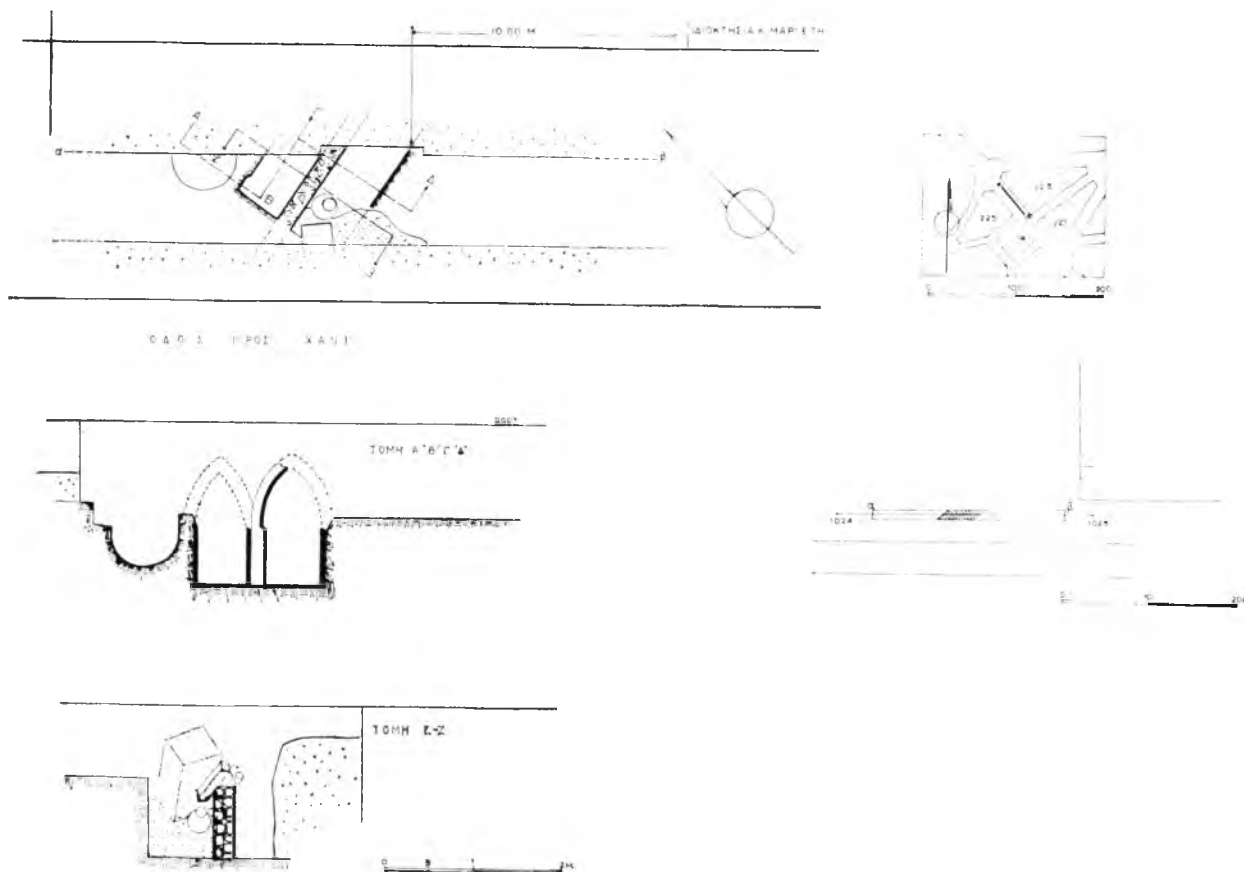
Σχέδ. 16. Μέγαρο. Πλατεία 'Αγ. 'Ιωάννου Γαλιλαίου (Ο.Τ. 226). Τοπογραφικὸν σχεδιογράφημα περιοχῆς, κάτοψις καὶ τομαὶ άνασκαφῆς
