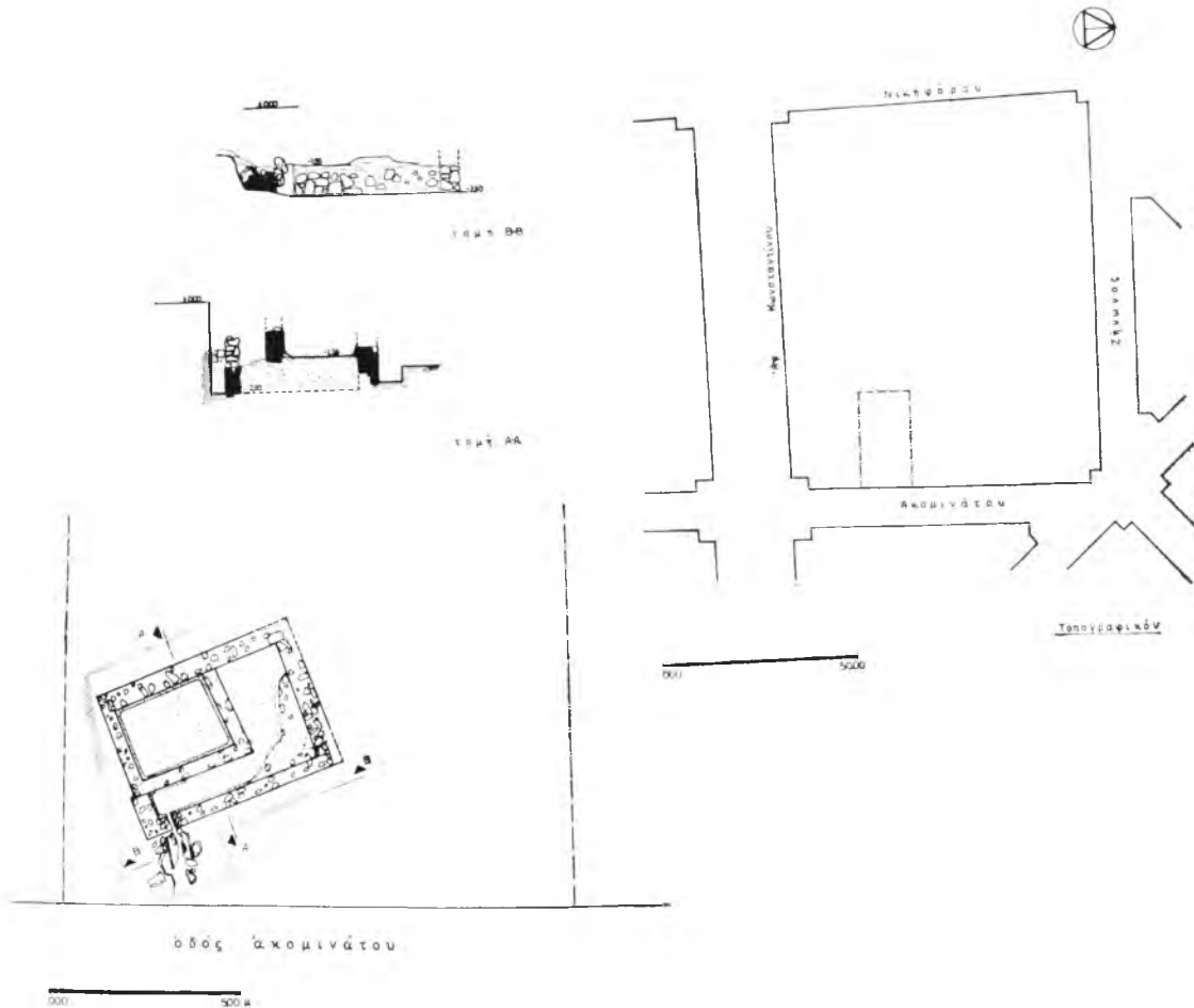
Σχέδ. 2. Τοπογραφικὸν διάγραμμα, κάτοψις καὶ τομαὶ ἀνασκαφῆς ἐπὶ τῆς ὁδοῦ Ἀκομινάτου 12
