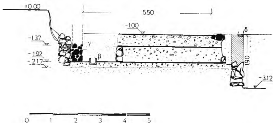
Σχέδ. 5. Ἐλευσίς. Τομή τῆς Ἱερᾶς ὁδοῦ, ἀποκαλυφθείσης παρὰ τὴν Ἱεράν ὁδὸν 8
