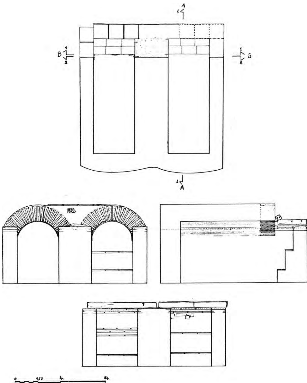
Σχέδ. 2. Νέα Αγχιάλος. Οικόπεδο Χρ. Ρίζου. Κάτοψη και τομές των καμαροσκέπαστων τάφων 216, 217.
