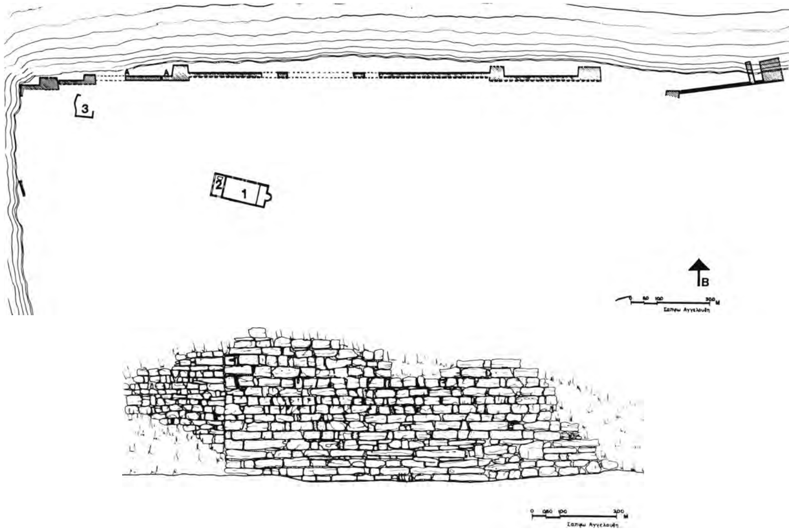
Σχέδ. 2. Λήμνος. Κότσινας. Κάτοψη του μεσαιωνικού φρουρίου και αποτύπωση της βορινής πλευράς.
