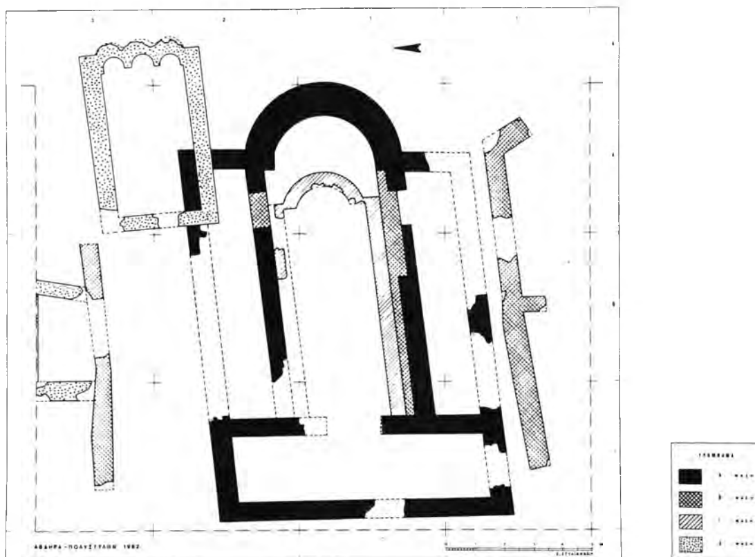
Σχέδ. 3. Πολύστυλον (Αβδηρα). Κάτοψη τρίκλιτης βασιλικής και μεταγενέστερων φάσεων (αποκατάσταση).
