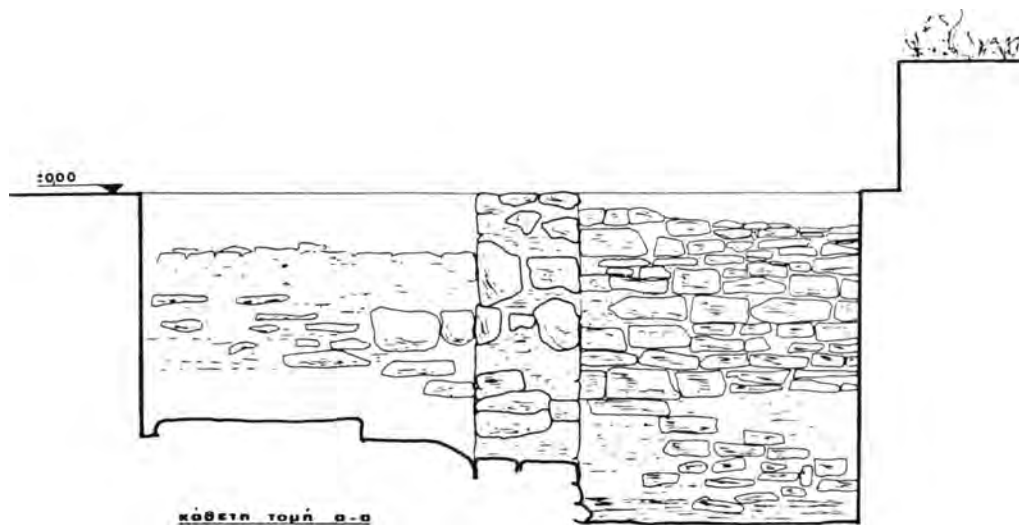
Σχέδ. 2. Λιμένας Θάσου. Οικόπεδο Απ. Γεωργαλή. Τομή δρόμου και τοίχου Τ ΙΙ.
