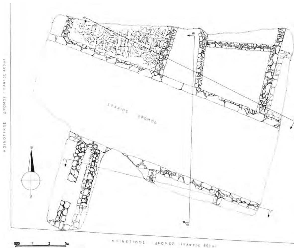
Σχέδ. 2. Καλλιθήρο. Οικόπεδο Γ. Λαγού. Κάτωψη του αρχαίου δρόμου.
