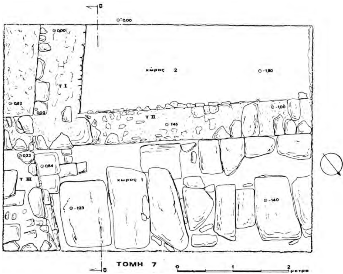
Σχέδ. 1. Λιμένας Θάσου. Οικόπεδο Απ. Γεωργαλή. Τμήμα ρωμαϊκού δρόμου με αγωγό και τοίχο κτιρίου.
