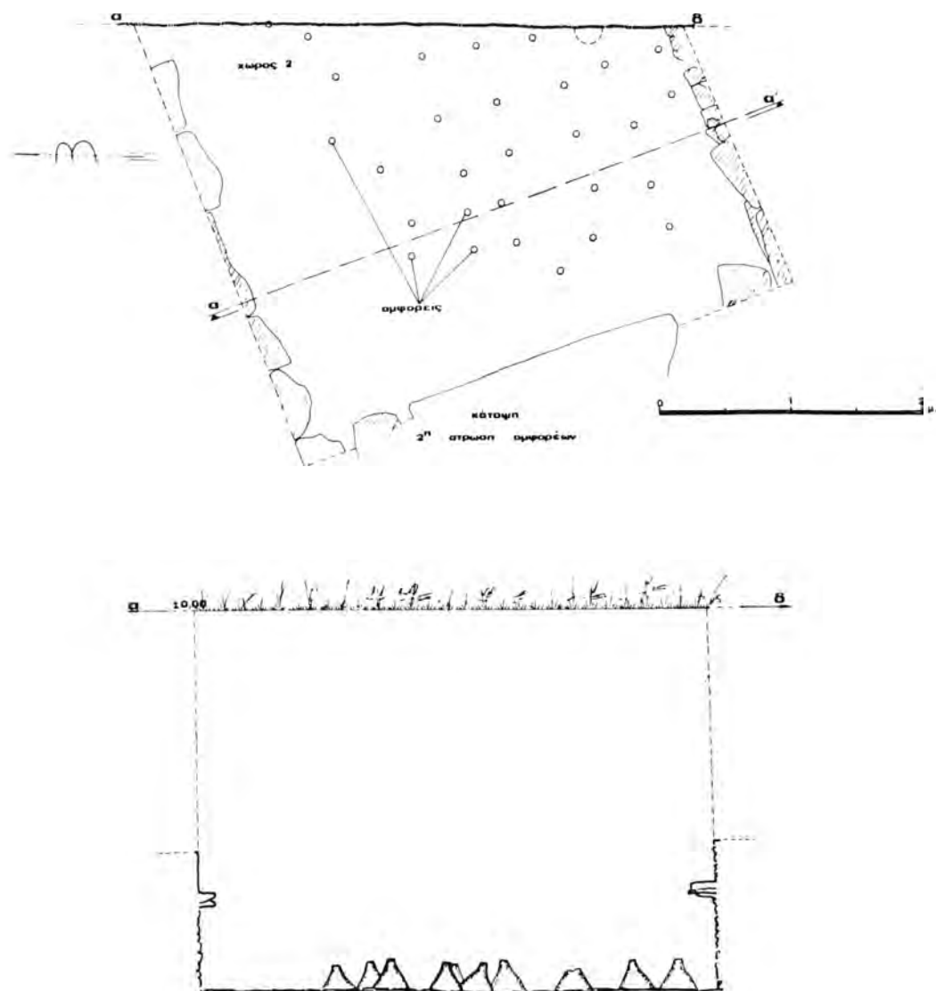
Σχέδ. 4. Λιμένας Θάσου. Οικόπεδο Γ. Μαγαφίνη. Κάτοψη χώρου 2 με αμφορείς για αποστράγγιση και τομή α-α'.
