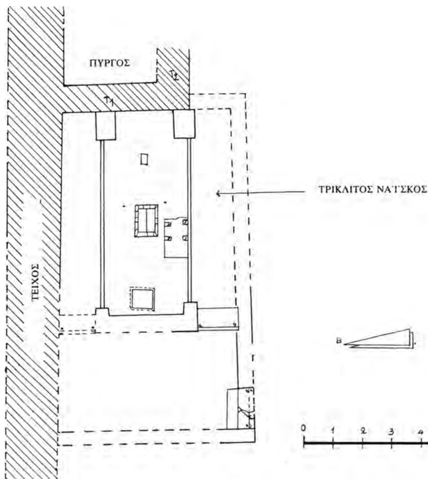
Σχέδ. 1. Νέα Αγχιάλος. Οικόπεδο Παπαγρηγορίου. Κάτοψη τμήματος του οχυρωματικού τείχους και τρίκαιτος ναῖσκος.
