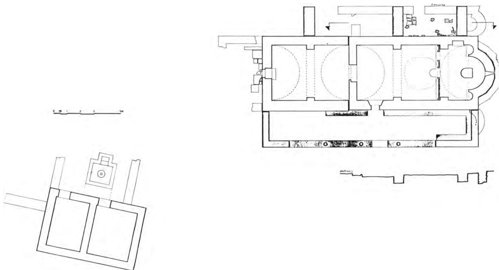
Σχέδ. 4. Νέα Σαμψούντα Πρέβεζας. Μονή Κοιμήσεως Θεοτόκου στο Κοζίλι. Κάτοψη του καθολικού και των προσκτισμάτων.
