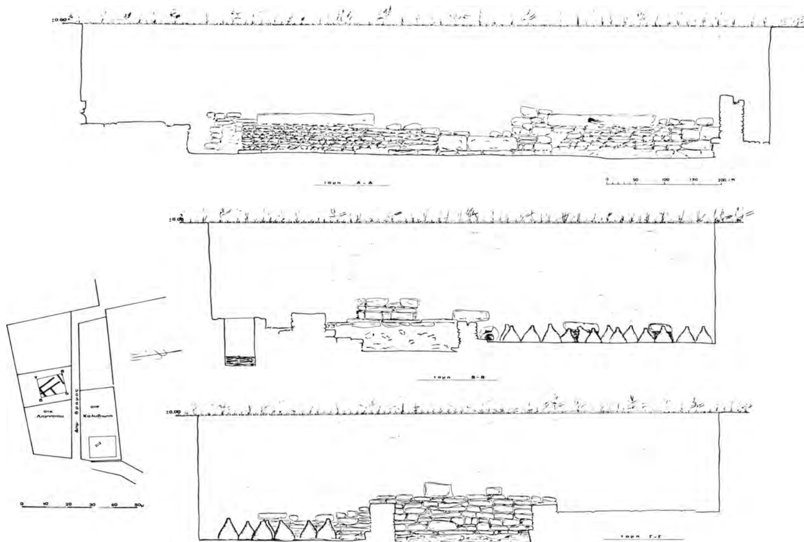
Σχέδ. 5. Λιμένας Θάσου. Οικόπεδο Γ. Μαγγαφίνη. Τομή Α-Α' χώρου 3 και τομή Β-Β' με υπερυψωμένο αποστραγγιστικό σύστημα.
