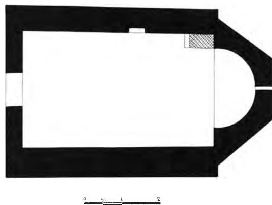
Σχέδ. 1. Ρόδος. Μαρितσά. Ἅγιος Γεώργιος. Κάτοψη του ναυδρίου.
