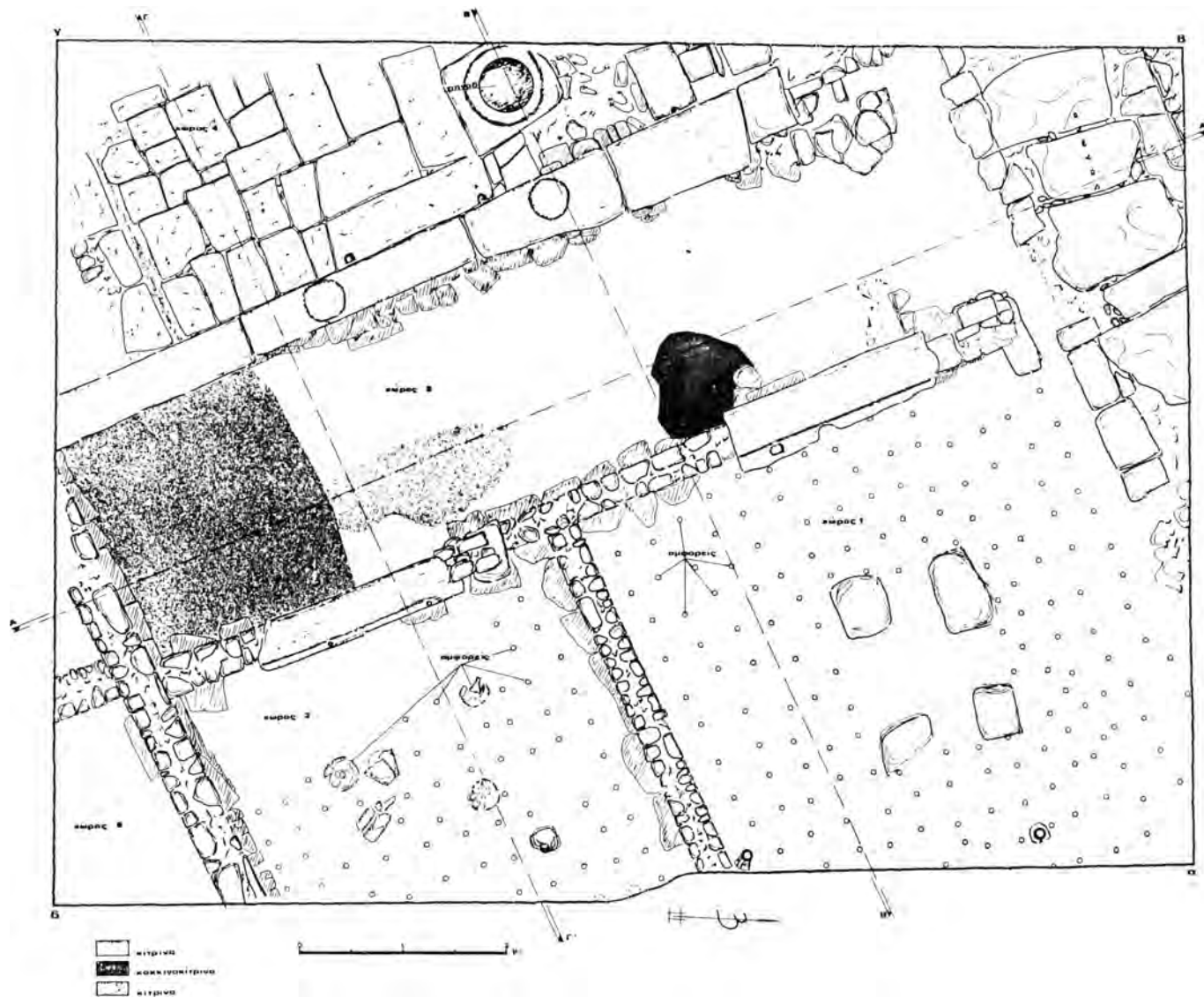
Σχέδ. 3. Λιμένας Θάσου. Οικόπεδο Γ. Μαγκαφίνη. Κάτοψη της ανασκαφής.
