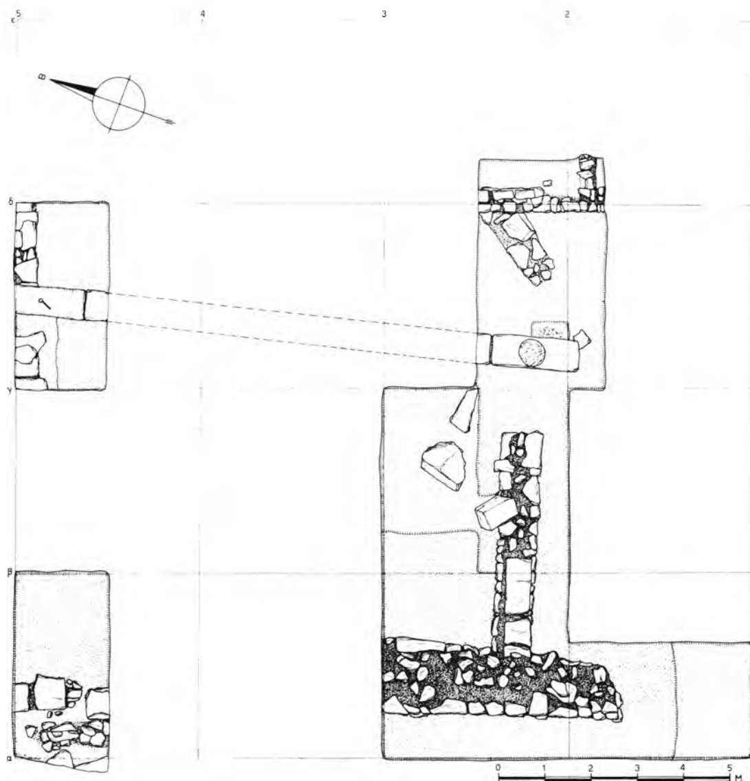
Σχέδ. 1. Θέση «Μπας-Μπαξέ». Οικόπεδο Ιω. Σαμαρά. Κάτοψη της ανασκαφής.
