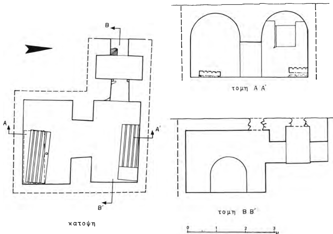
Σχέδ. 2. Φίλιπποι-Κρηνίδες. Ανατολικό νεκροταφείο. Δίδυμος τάφος στο αγροτεμάχιο αριθ. 461.
