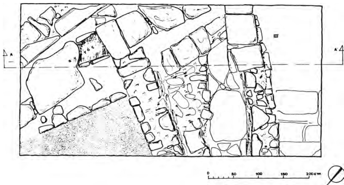
Σχέδ. 8. Λιμένας Θάσου. Οικόπεδο Ευστρ. Πυρήνα. Κάτοψη τομής Δ.
