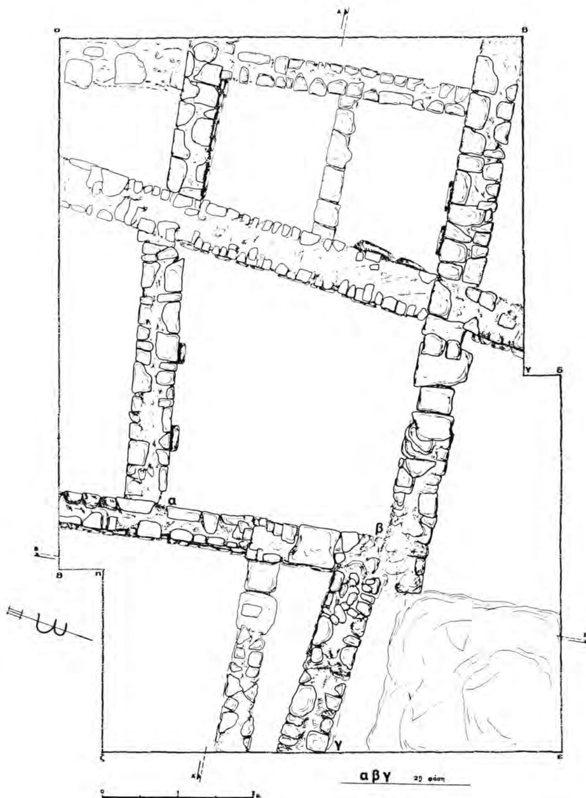
Σχέδ. 9. Λιμένας Θάσου. Οικόπεδο Ιφ. Ράνη. Κάτοψη της ανασκαφής.
