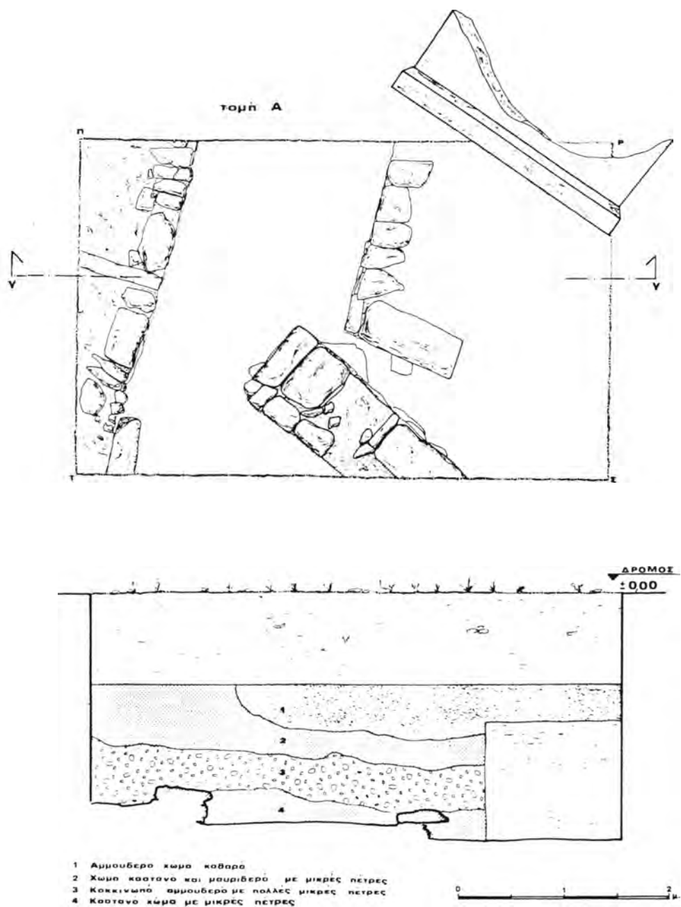
Σχέδ. 12. Λιμένας Θάσου. Οικόπεδο Θ. Βασιλάκου. Κάτοψη τομής Α και στρωματογραφία γ-γ.
