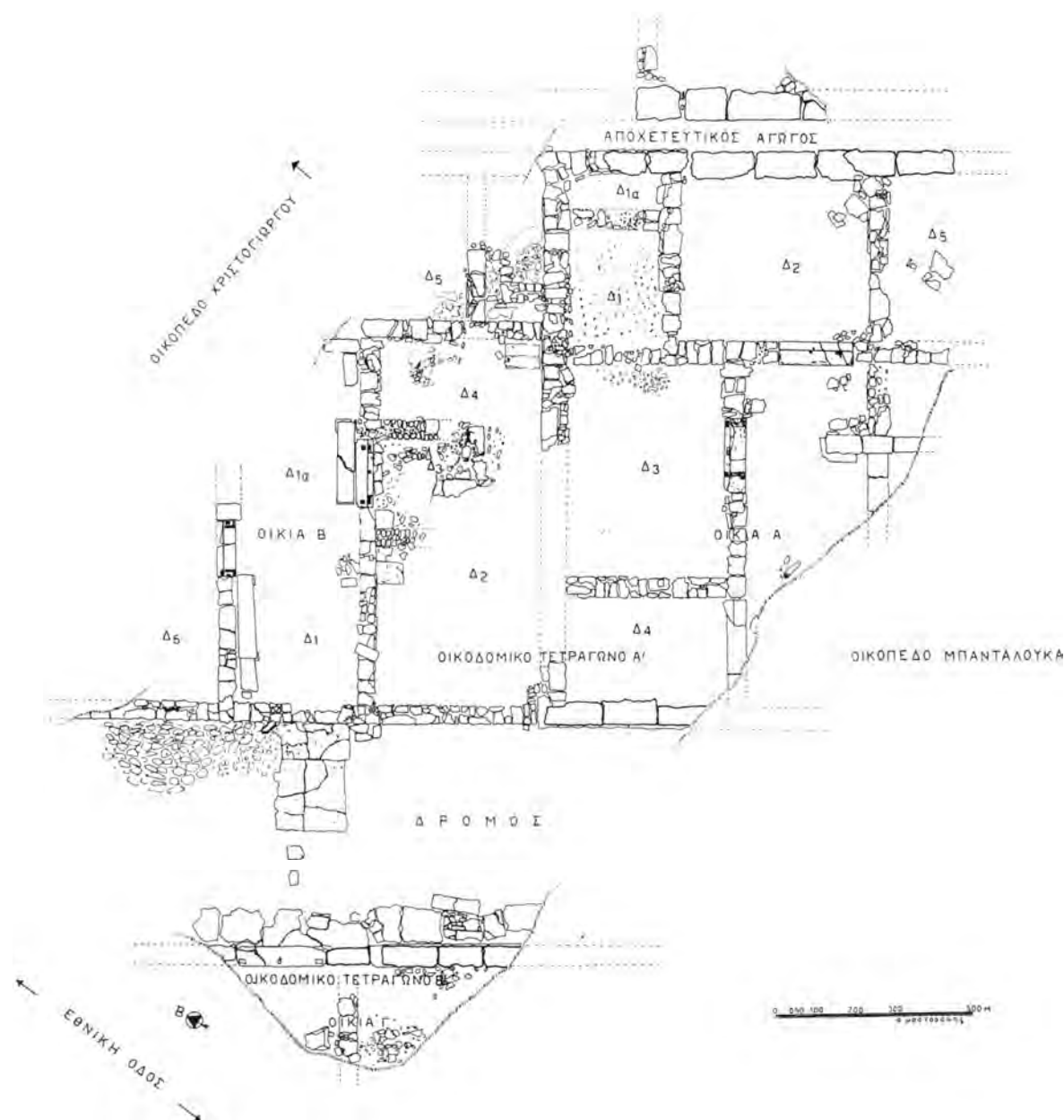
Σχέδ. 1. Άρτα. Οικόπεδο Ζήκου. Κάτοψη της ανασκαφής.
