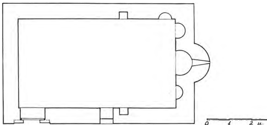
Σχέδ. 5. Προμύριον Πηλίου. Κάτωψις του ναού των Ἀγίων Ἀποστόλων.
