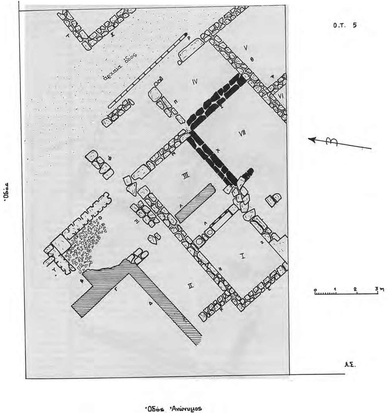
Σχέδ. 3. Χαλκίδα. Οἰκόπεδο Γιαμᾶ. Κάτοψη τῆς ἀνασκαφῆς.
