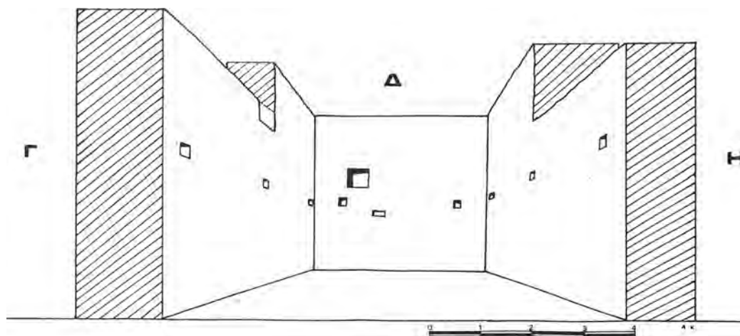
Σχέδ. 6. Χαλκίδα. Οικόπεδο Μπασούκου. Τομή του αποθέτη (δωμ. 1).
