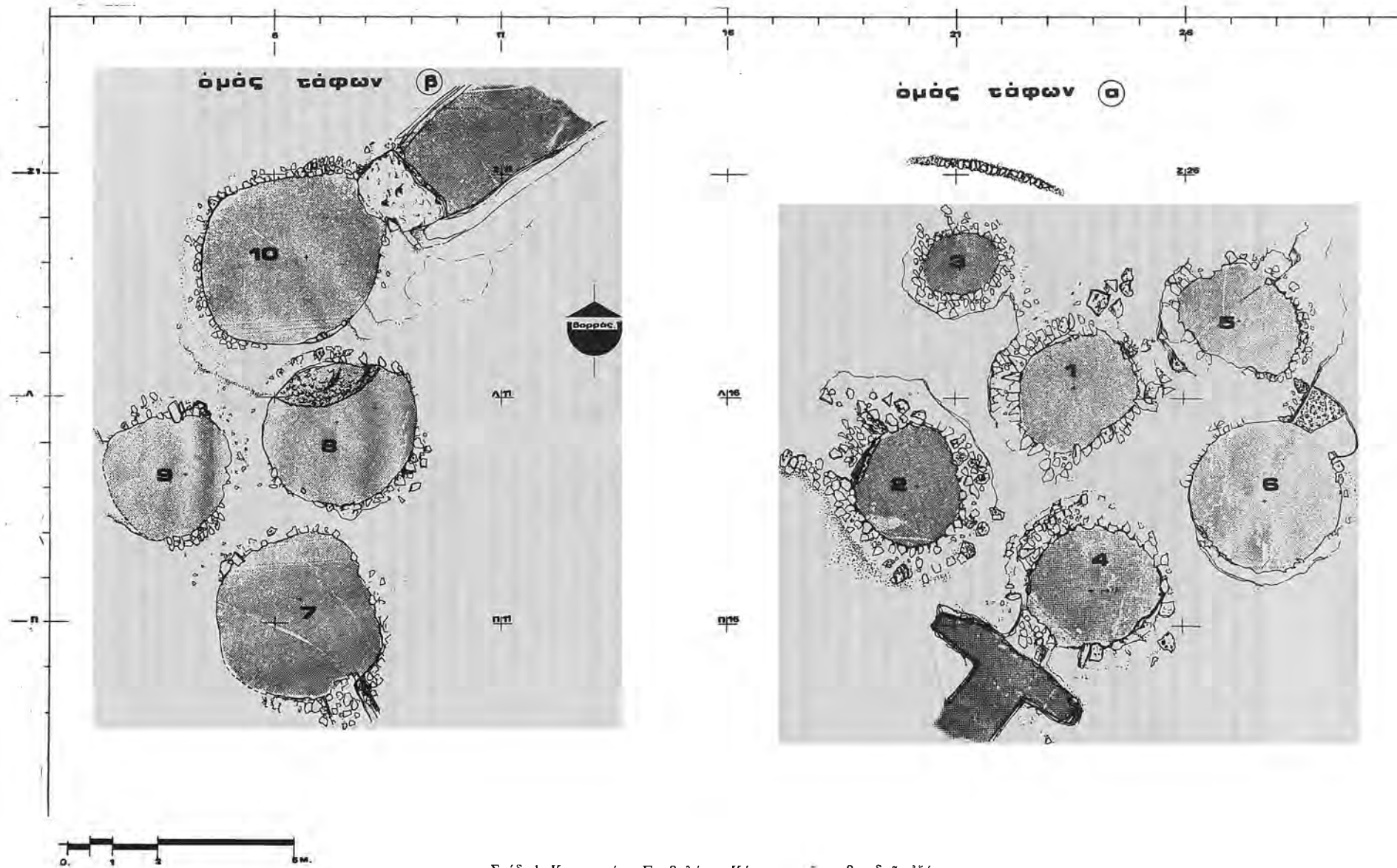
Σχέδ. 1. Κουκουνάρα-Γουβαλάρη. Κάτοψις τοῦ τυμβοειδοῦς ἐξάρματος α.
