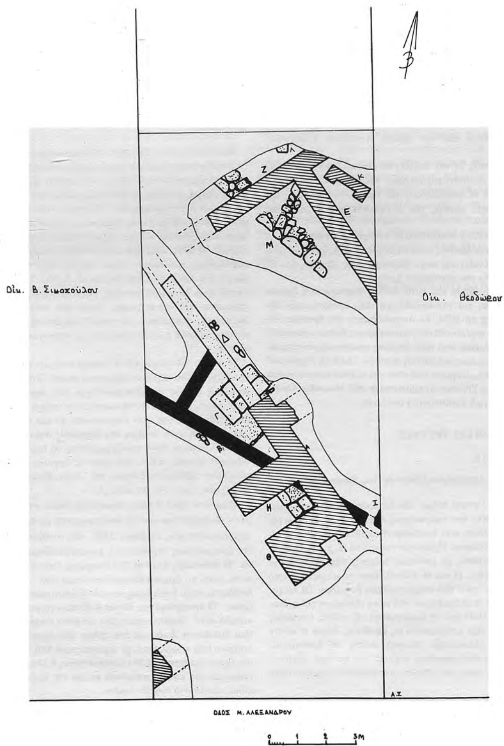
Σχέδ. 1. Χαλκίδα. Οικόπεδο Κατσιαβέλου. Κάτοψη της ανασκαφής.
