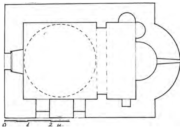
Σχέδ. 4. Προμύριον Πηλίου. Κάτωψις του ναού της Ἁγίας Παρασκευῆς.
