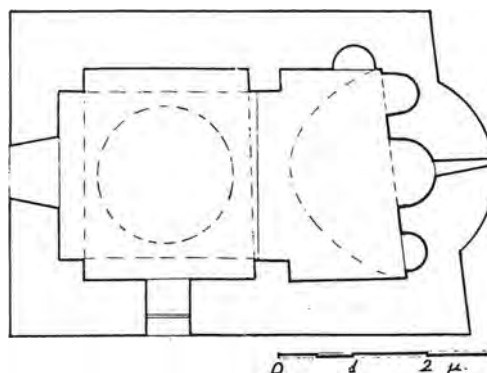
Σχέδ. 1. Προμύριον Πηλίου. Κάτωψις τοῦ ναοῦ τοῦ Γενεσίου Θεοτόκου εἰς Μουδσγες Πλατανιάς.
