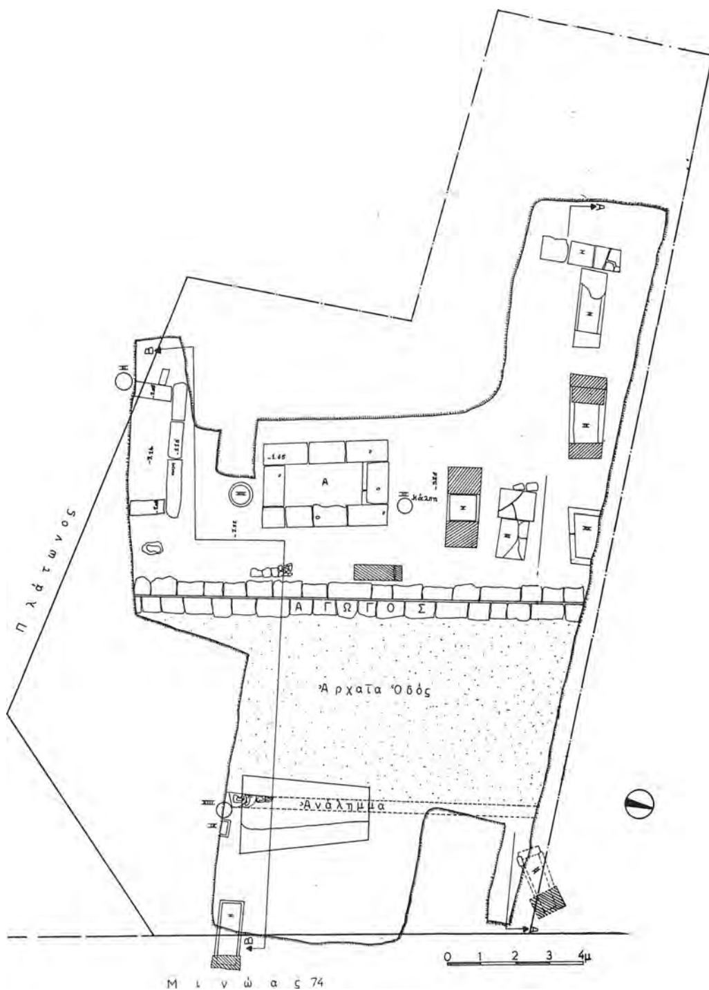
Σχέδ. 12. Μέγαρο. Όδος Μινώας 74 καί Πλάτωνος. Κάτοψη της ανασκαφής.
