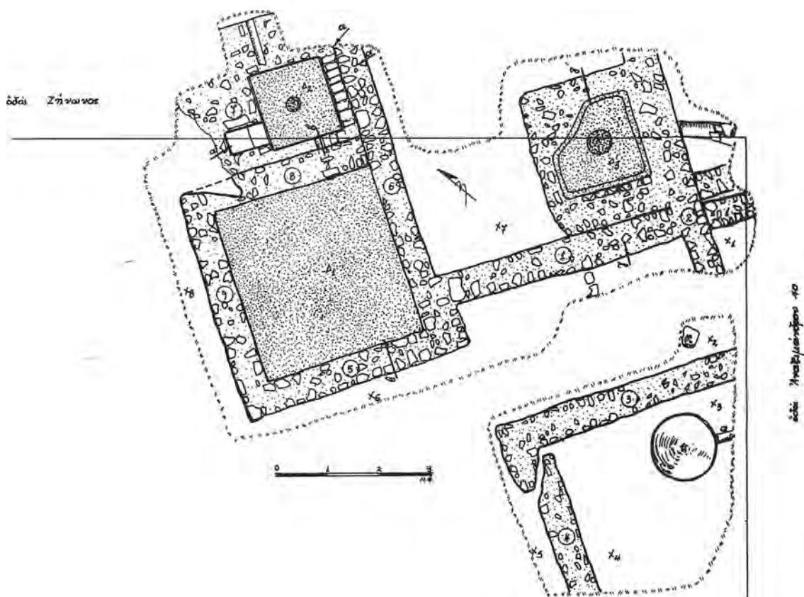
Σχέδ. 7. Πάτρα. 'Οδός' Αναξιμάνδρου 40. Κάτοψη της ανασκαφής.
