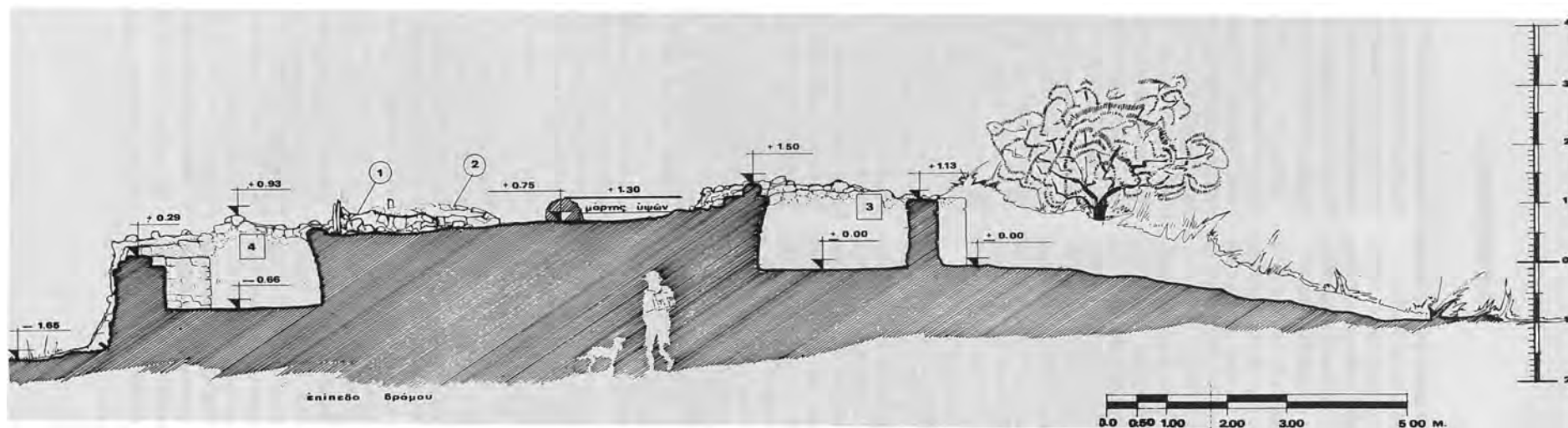
Σχέδ. 4. Τομή του τύμβου Καμινίων.
