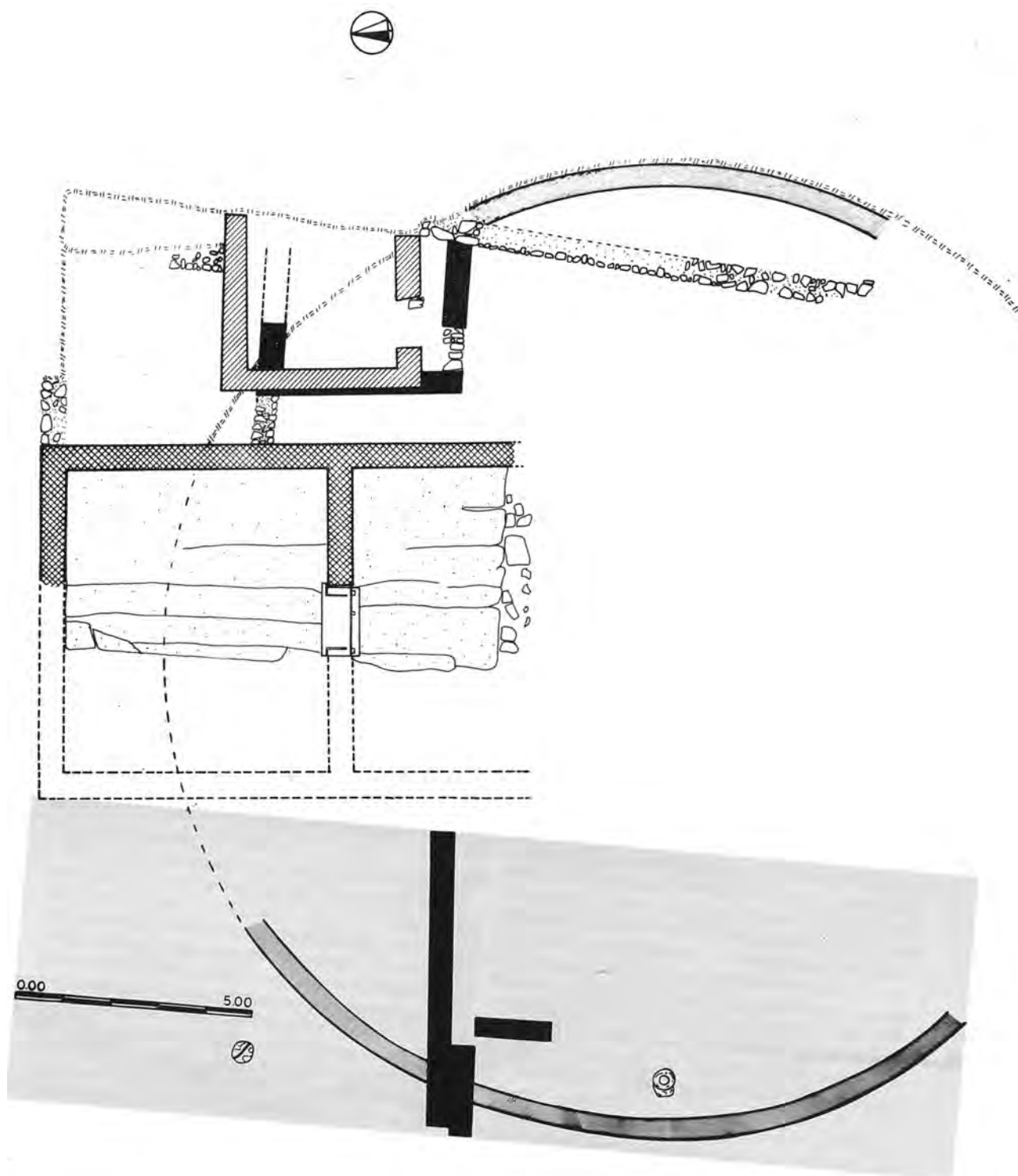
Σχέδ. 2. Καμάριζα. Θέση Πουσιπέλια. Οι δύο φάσεις της ανασκαφής.
