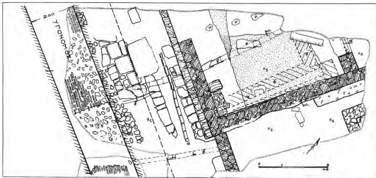
Σχέδ. 2. Πάτρα. 'Οδός Γούναρη 48. Κάτοψη της ανασκαφής.
