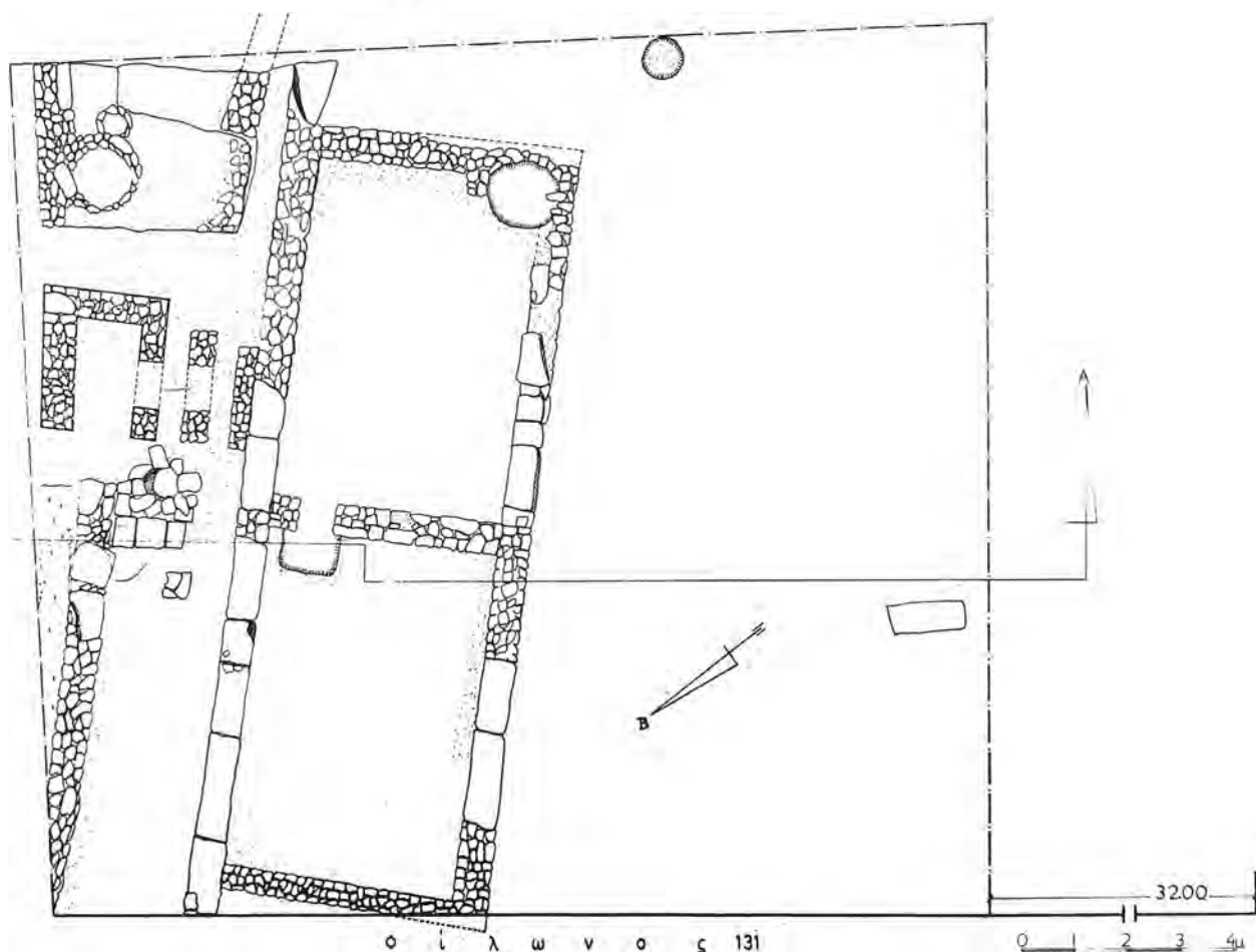
Σχέδ. 8. Πειραιάς. Ὁδὸς Φίλωνος 131. Κάτοψη τῆς ἀνασκαφῆς.
