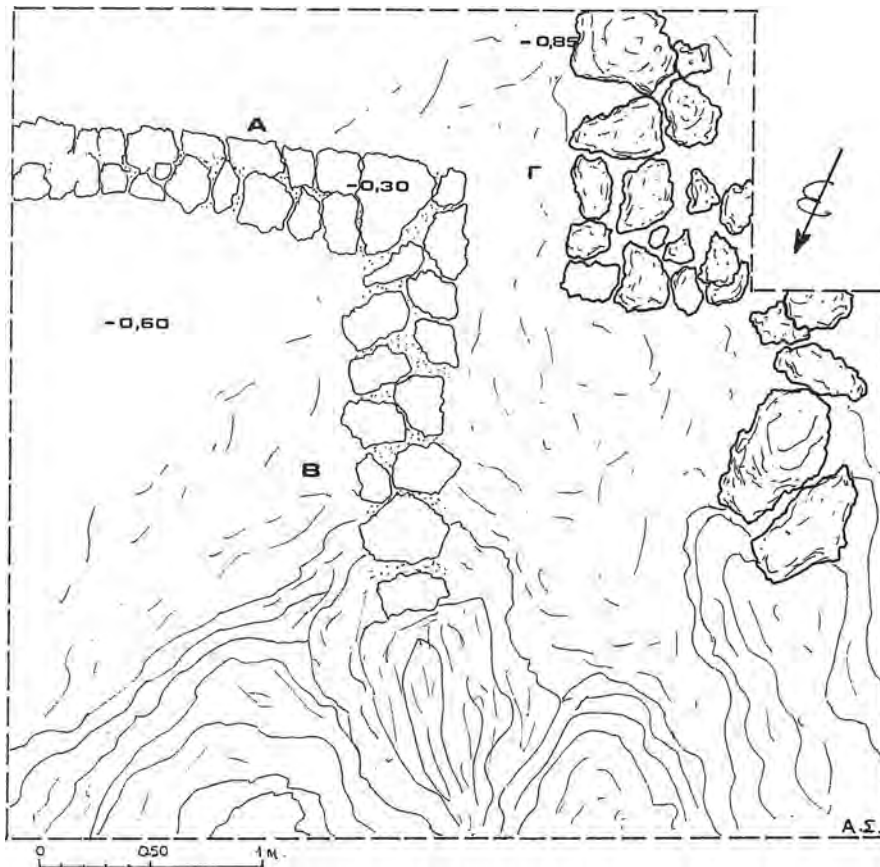
Σχέδ. 7. Βάρκα Ψαχνών. Κάτοψη της τομής Ι.
