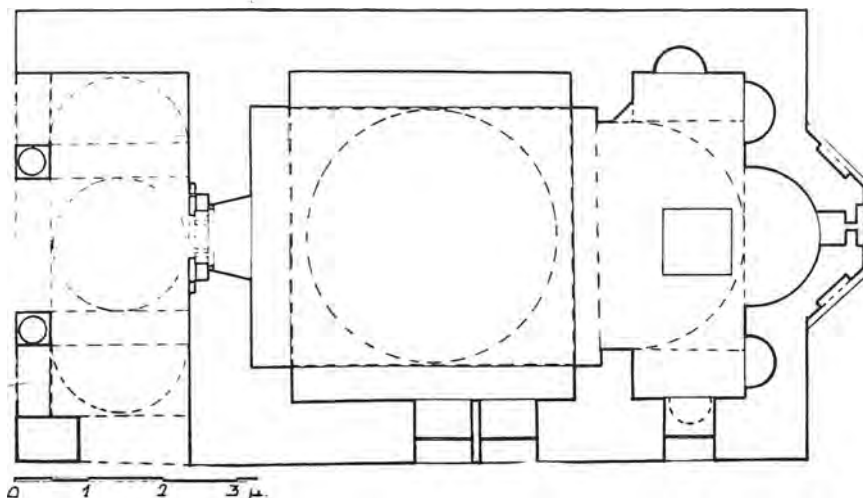
Σχέδ. 2. Προμήριον Πηλίου. Κάτοπις τοῦ ναοῦ τῆς Ἁγίας Τριάδος.
