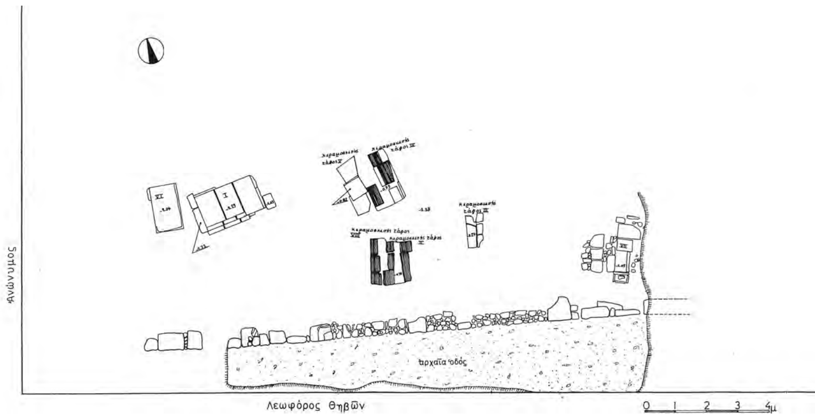
Σχέδ. 9. Ἐλευσίνα. Λεωφόρος Θηβών (Ο.Τ. 156). Κάτοψη τῆς ἀνασκαφῆς.
