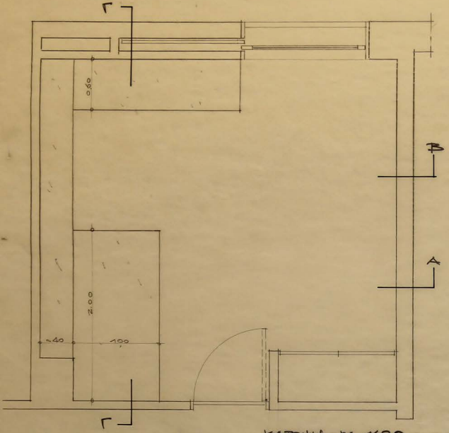
ΚΑΤΩΛΙΣ Κ. 1/20
