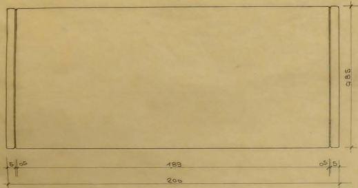
ΚΑΤΩΦΛΙΣ ΕΛ. 1/10
