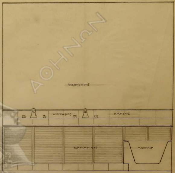
τομή Β-Β
