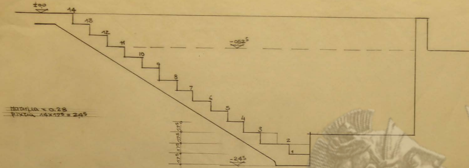
Τομή α-α κλίμακας 1/20
