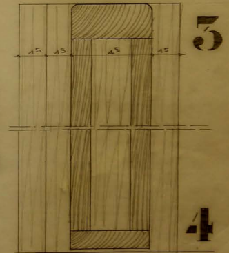
ΚΑΤΑΚΟΡΥΦΗ ΤΟΜΗ ΚΑΙΝΑΣ 1/21
