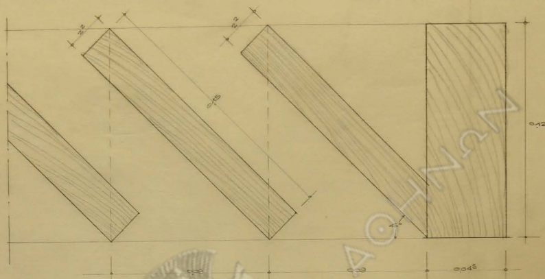
ΛΕΠΤ. ΟΡΙΖΟΝΤΙΑ ΤΟΜΗ ΚΑΙΝΑΣ
