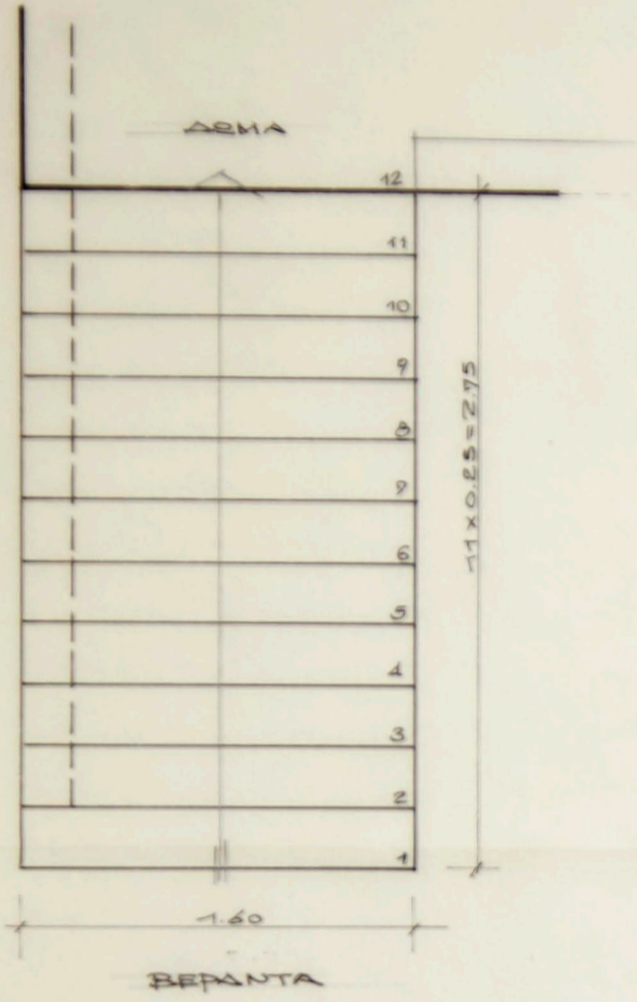
ΚΑΤΟΨΙΣ ΚΛ. 1/20
