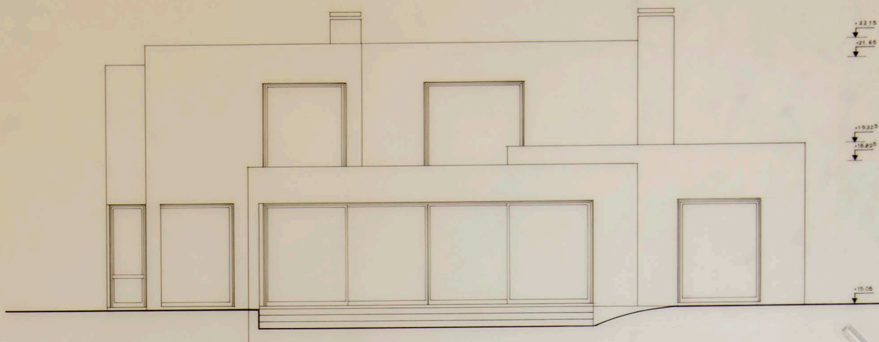
Οψη ΝΟΤΙΑ
