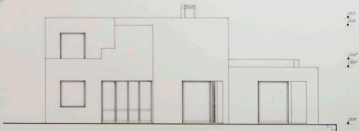
Οψη ΔΥΤΙΚΗ
