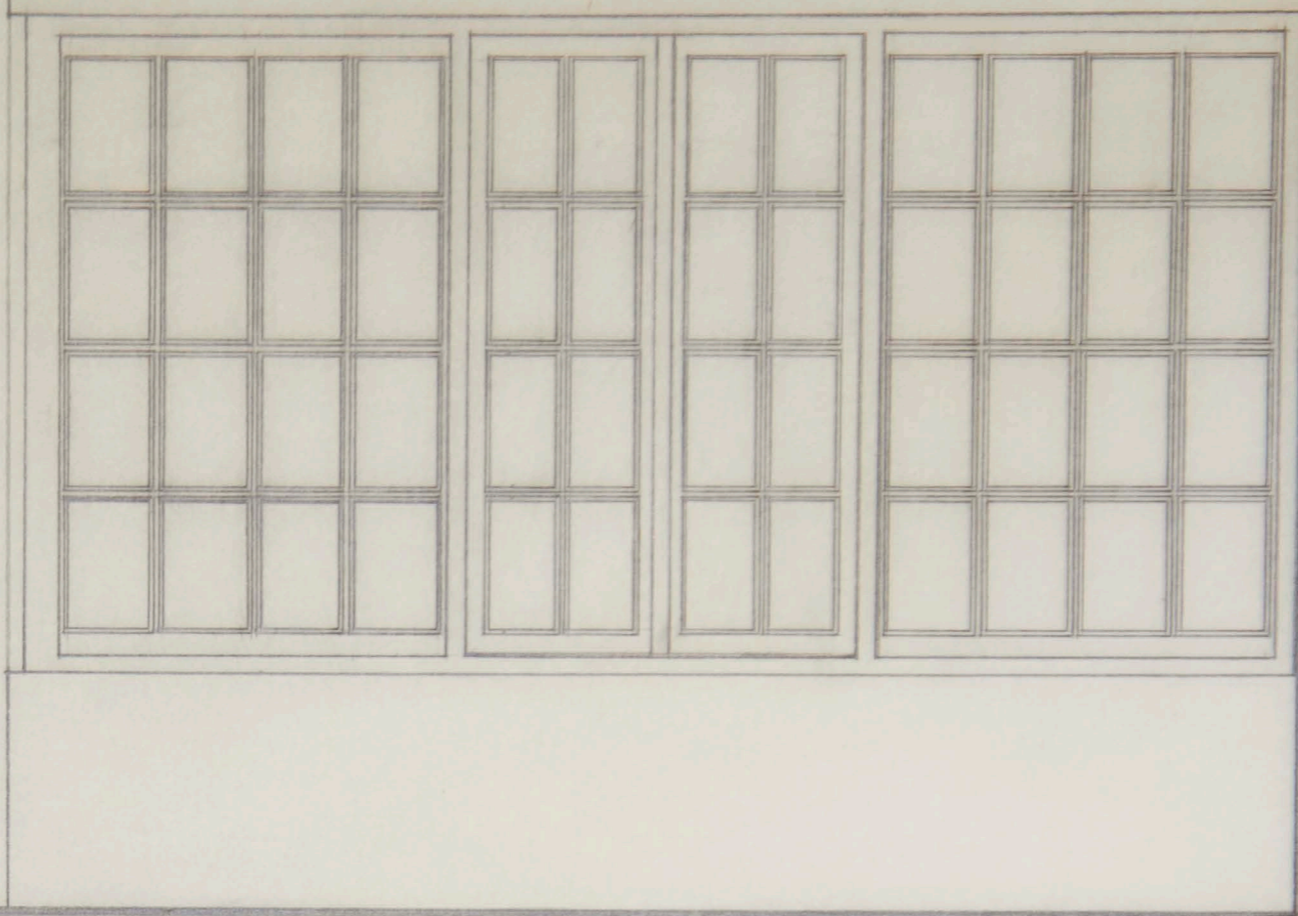
ΚΥΡΙΑ ΟΨΗ ΤΖΑΜΑΡΙΑΣ ΣΑΛΟΝΙΟΥ - ΚΛΙΜΑΚΑ 1:20
