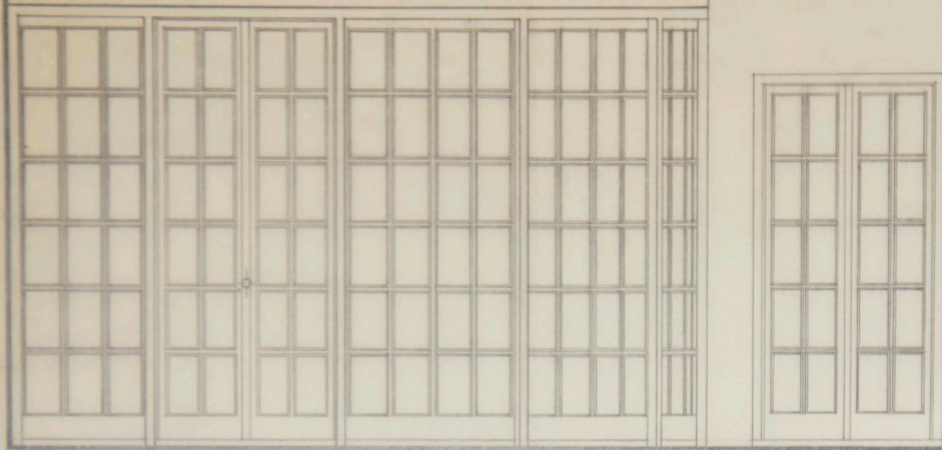
ΟΨΗ ΤΖΑΡΑΡΙΑΣ ΤΡΑΠΕΖΑΡΙΑΣ - ΚΙΜΑΚΑ 1:20
