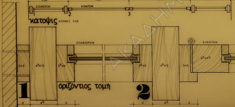
οφίς ΚΛΙΜΑΞ 1:10
