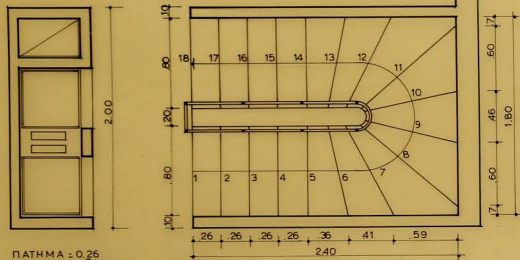
ΠΑΤΗΜΑ + 0.26 ΡΙΧΤΥ = 1x17.3 = 3.10 κάτοψις ορόφου
