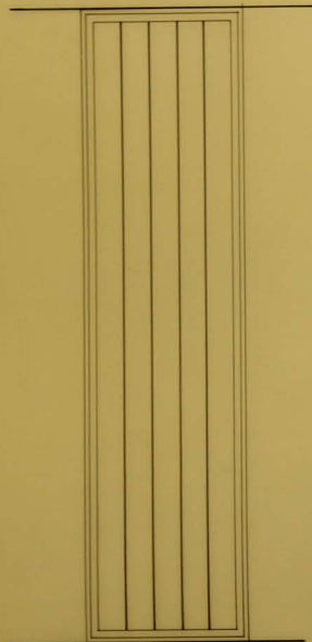
όψις εξωτερική ΚΛΙΜΑΞ 1:10
