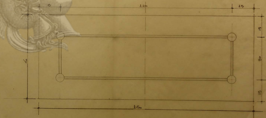
κατοψη κολωνος 1:5
