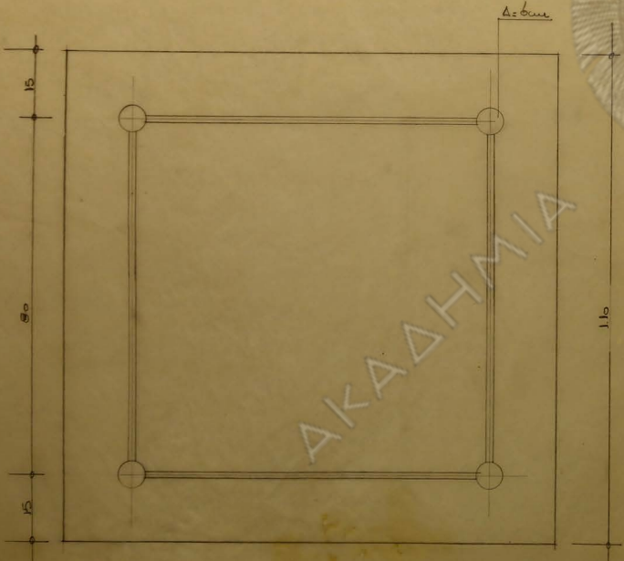
οψη κολωνος 1:5
