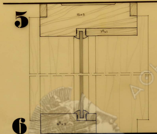
κατακόρυφος τομή σταθερού φύλλου
