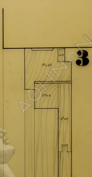
κατακ. τομή ΚΛΙΜΑΞ 1:1
