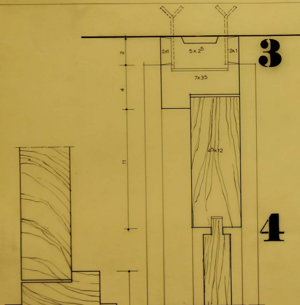
κατακόρυφος τομή ΚΑΙΜΑΣ 1:1
