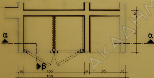
κατοψίς
