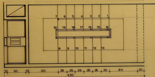
ΠΑΤΗΜΑ - 0.26 ΡΙΧΤΥ 17x20 = 3.40 κάτοψις ισόγειου
