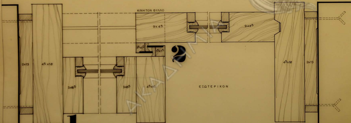
οριζόντιος τομή
