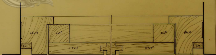
1 κλιμαξ 1:1 οριζ. τομή
