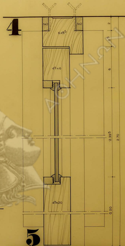
κατακόρυφος τομή θύρας
