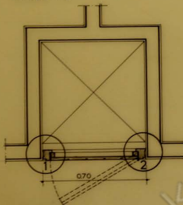
κάτοψις ΚΛΙΜΑΞ 1:10
