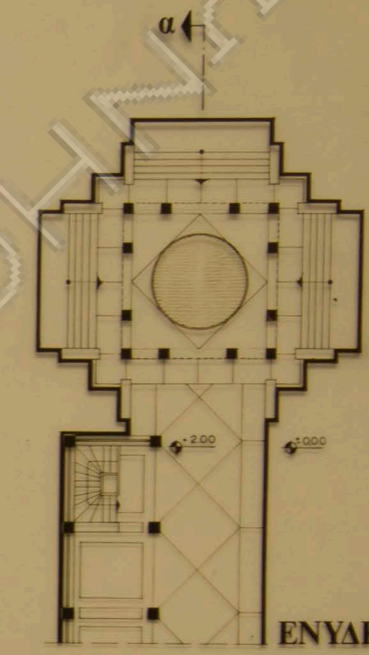
ΚΑΤΩΗ ΙΣΟΓΕΙΟΥ ΚΑ. 1:100
