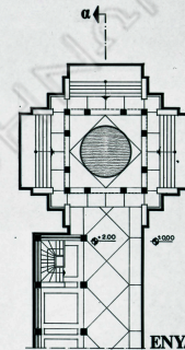
ΚΑΤΩΝ ΙΣΟΓΕΙΟΥ ΚΑ.1:100
