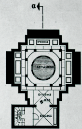
ΚΑΤΩΝ ΥΠΟΓΕΙΟΥ ΚΑ.1:100
