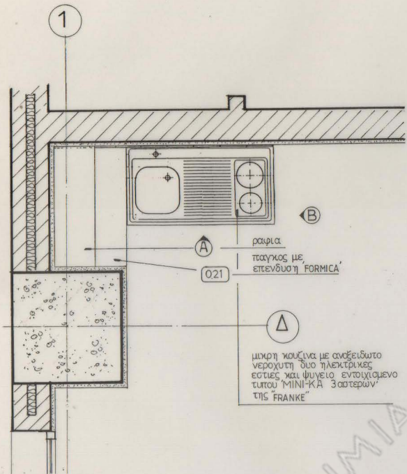
ΚΑΤΩΨΗ ΚΛ.1:20
