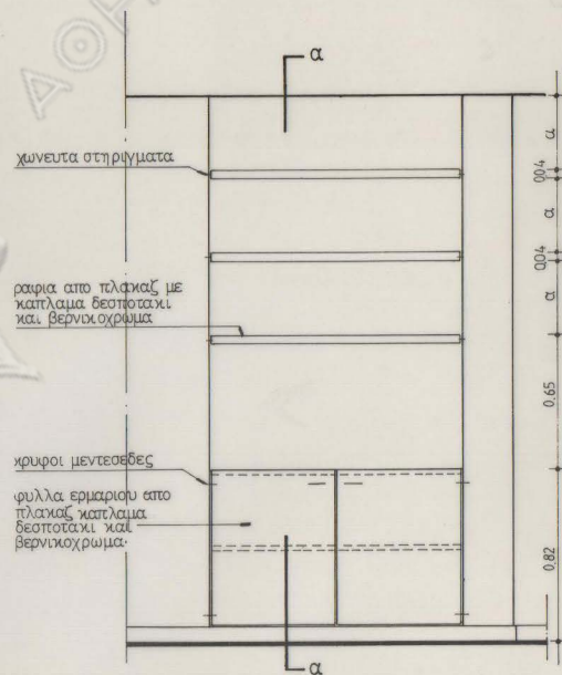
ΟΨΗ ΚΛ. 1:20
