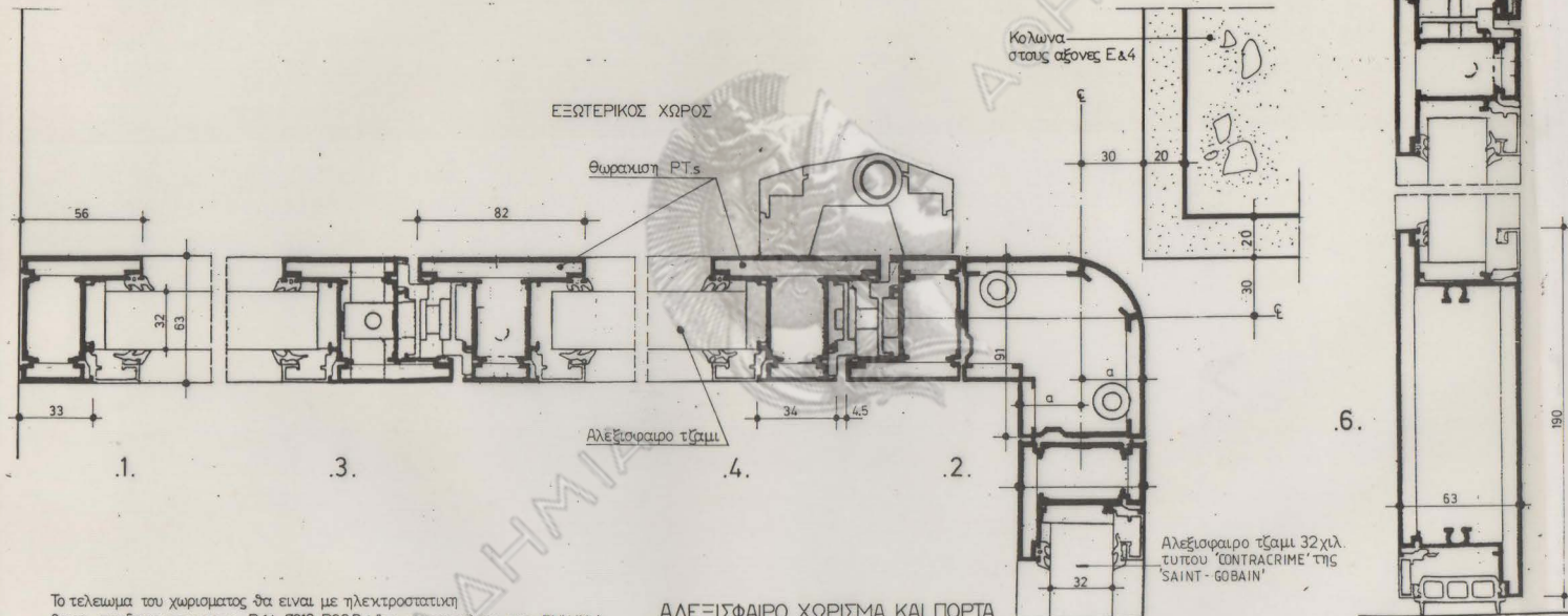
ΤΟΜΗ ΣΤΗ ΠΟΡΤΑ
