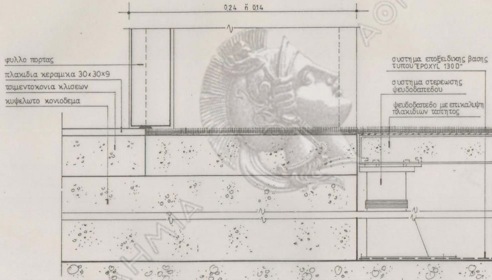
1. Λεπτομέρεια στην είσοδο προς χώρους υγιεινής κλπ Ισογείου, Α' και Β' ορόφου
