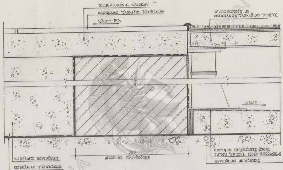
1. Λεπτομέρεια θύρας-χωφούς-0.06α, 0.45α και 0.69α
