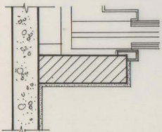
ΚΑΤΩΗ ΟΡΟΦΩΝ
