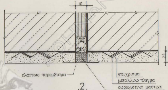
2. ΑΡΜΟΣ ΔΙΑΣΤΟΛΗΣ ΤΟΙΧΟΥ Α.Δ.Τ4
