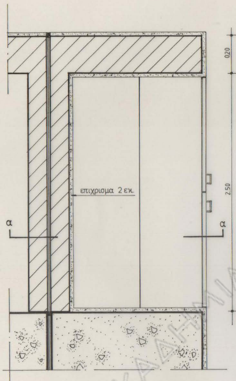
ΚΑΤΟΨΗ ΚΛ. 1:10
