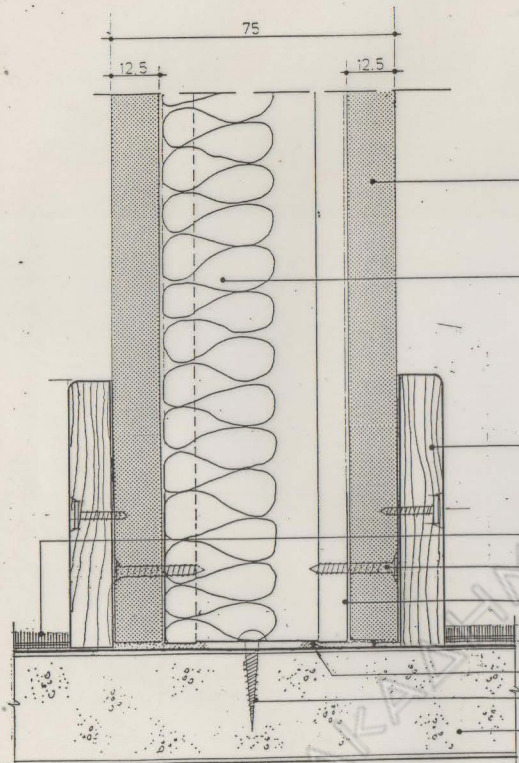
1. ΛΕΠΤΟΜΕΡΕΙΑ ΔΑΠΕΔΟΥ ΚΛ.1:1
