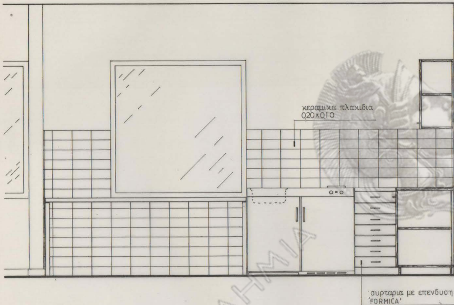
ΟΨΗ Α Κλ.1:20
