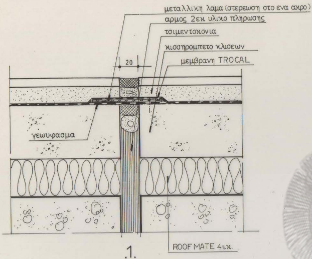
1. ΑΡΜΟΣ ΔΙΑΣΤΟΛΗΣΗΣ ΔΑΠΕΔΟΥ Α.Δ. Δ5
