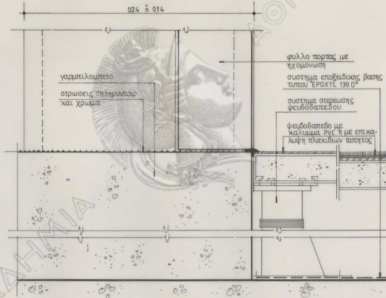
1. Λεπτομερεια στην εισοδο προς χωροσ κλιματισμου Ισογειου, Α' και Β' οροφου
