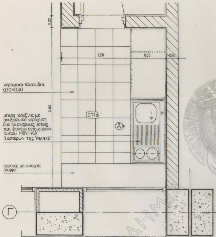
ΚΑΤΟΨΗ Κλ. 1:20
