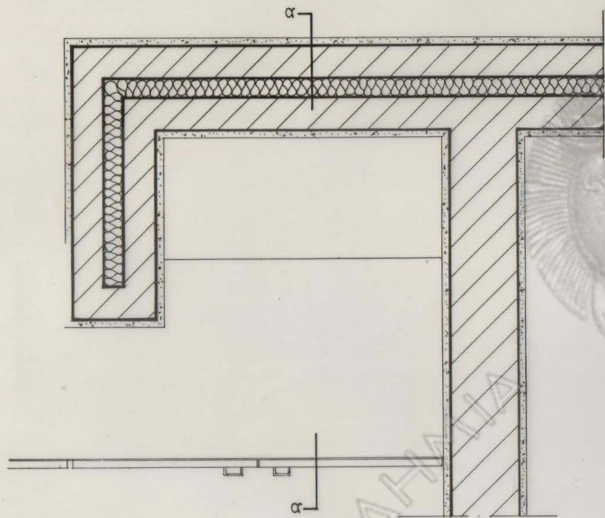
ΚΑΤΩΨΗ Κλ. 1:10
