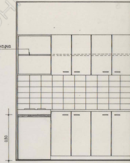
ΟΨΗ Β Κλ.1:20
