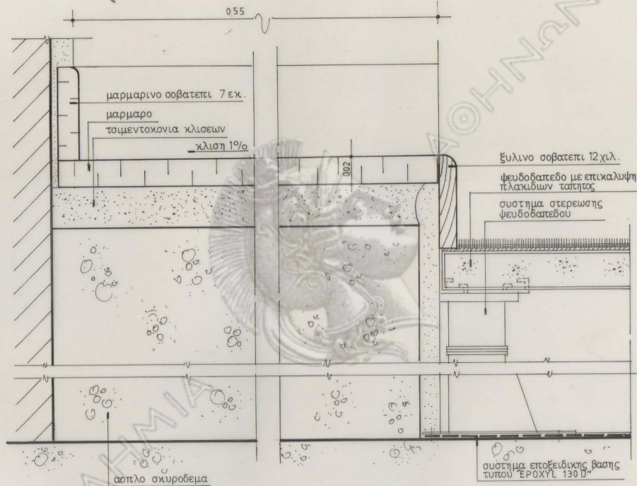
1. λεπτομερεια στους διαδρομους Α', Β' οροφου στην εσοχη εξω απο τους χωρους των W.C.
