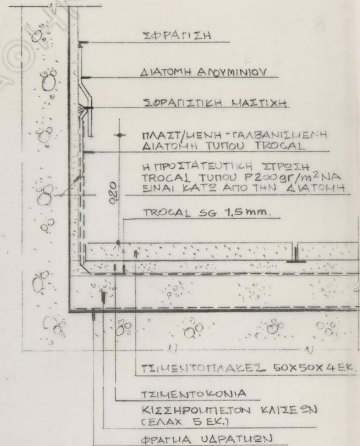
2. ΛΕΠΤ. ΒΟΗΘΗΤΙΚΟΥ ΚΤΙΡΙΟΥ.
