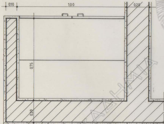
ΚΑΤΟΨΗ Κλ. 1:10
