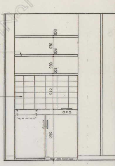
ΩΨΗ Α Κλ. 1:20
