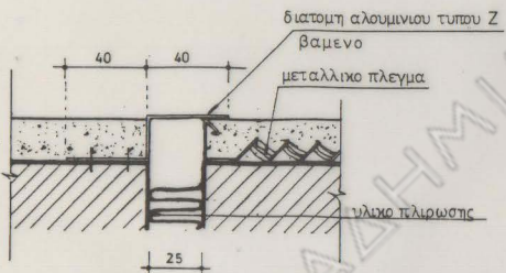
A.Δ.Τ.3
