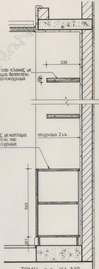
ΤΟΜΗ α-α Κλ. 1:10
