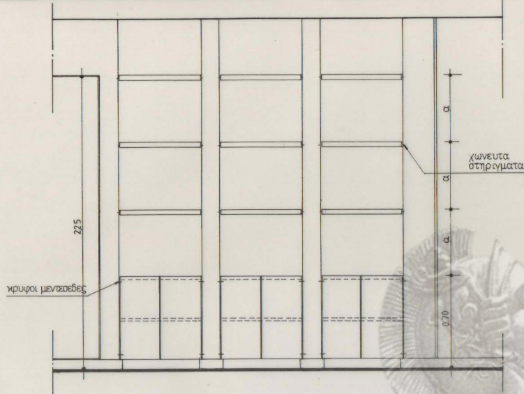
ΟΨΗ Κλ. 1:20
