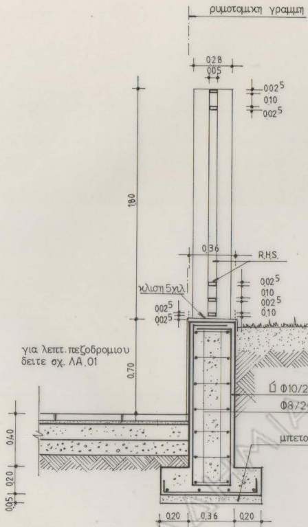
Α-Α ΤΟΜΗ ΣΤΗΝ ΠΕΡΙΦΡΑΣΗ
