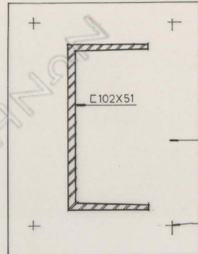
ΤΟΜΗ β'-β''
