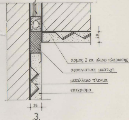
3. ΑΡΜΟΣ ΔΙΑΣΤΟΛΗΣ ΤΟΙΧΟΥ Α.Δ.Τ5
