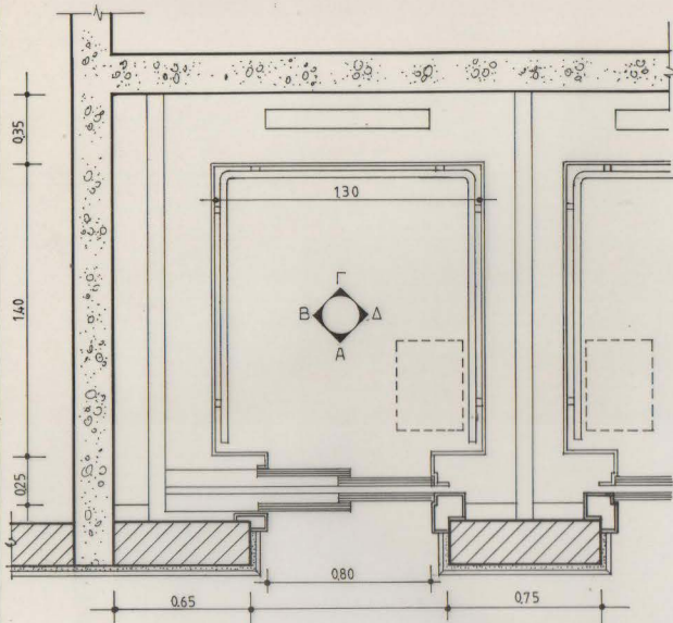
ΚΑΤΩΗ ΙΣΟΓΕΙΟΥ
