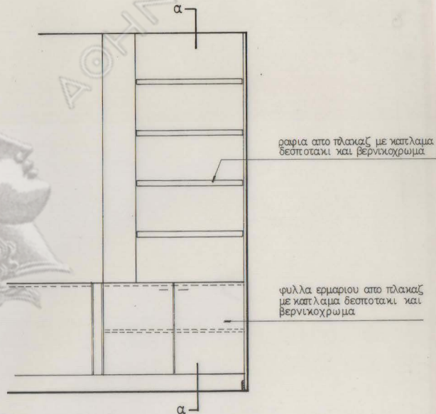
ΟΨΗ Κλ. 1:20
