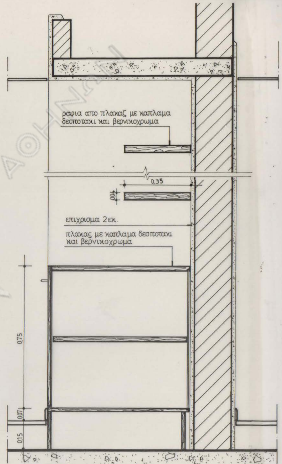
ΤΟΜΗ α α Κλ. 1:10
