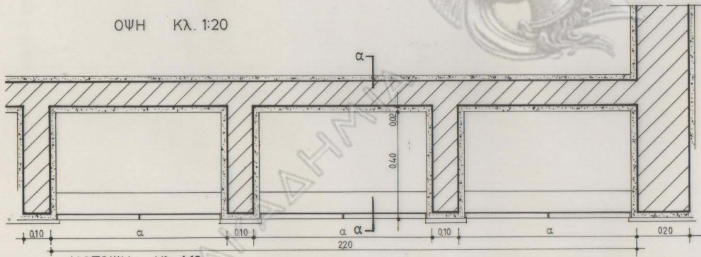
ΚΑΤΟΨΗ Κλ. 1:10
