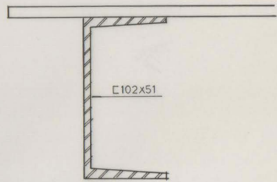
ΤΟΜΗ γ-γ''
