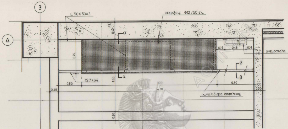
ΚΑΤΟΨΗ
