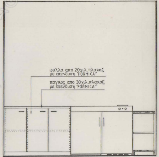
ΟΨΗ Α Κλ. 1:20
