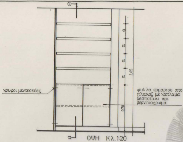
ΟΨΗ Κλ. 1:20
