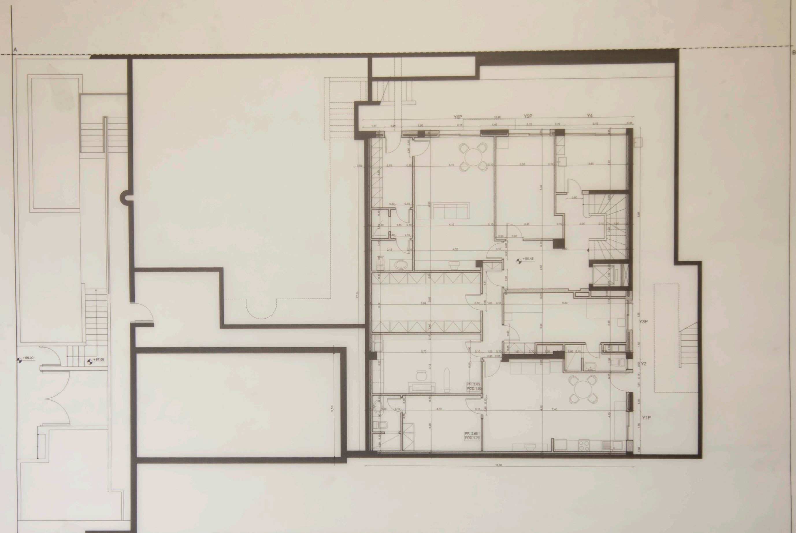
2. ΚΑΤΟΨΗ Α' ΥΠΟΓΕΙΟΥ
