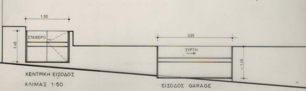
ΠΟΡΤΑ ΚΕΝΤΡ ΕΙΣΟΔΟΥ - ΟΥΗ ΚΛ. 1: 10
