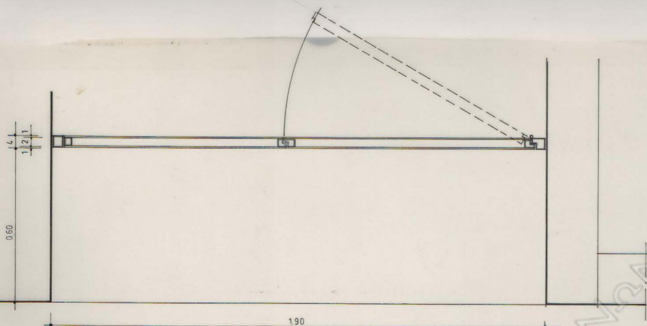
ΠΟΡΤΑ ΚΕΝΤΡ ΕΙΣΟΔΟΥ - ΚΑΤΩΗ ΚΛ. 1: 10
