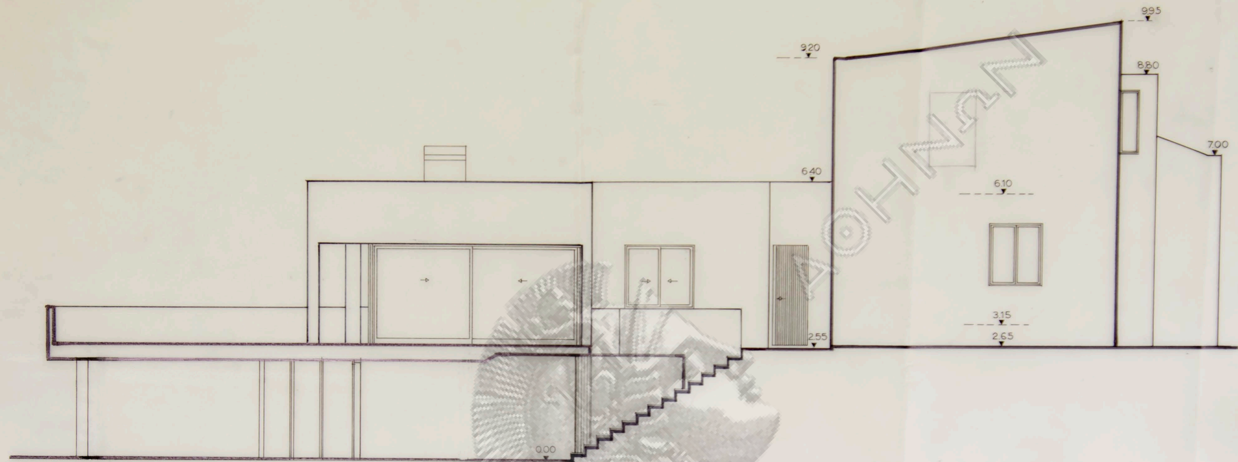
Οψη Ανατολική κλ. 1:50
