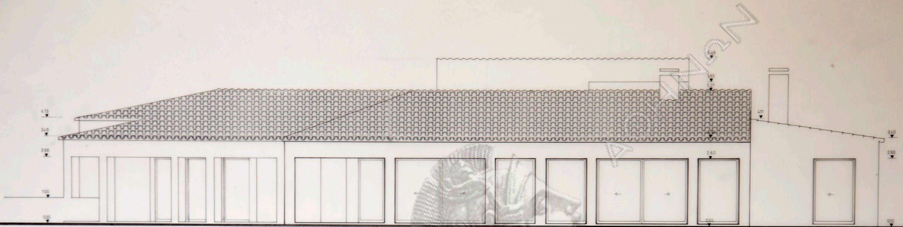
ΟΨΗ Ν.Α.
