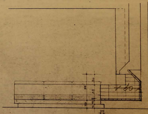
ΤΟΠΟΣ ΚΥΜΑΤΟΣ 1/20
