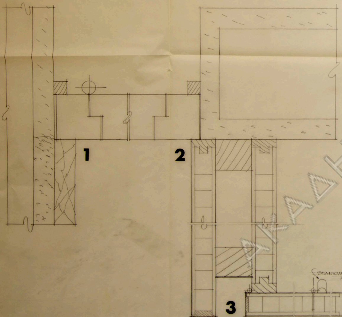
ΚΑΤΟΨΙΣ ΝΤΟΥΛΑΠΙΣΤΗ ΚΛ. 1:1
