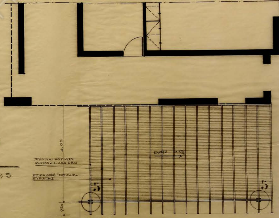
ΚΑΤΩΦΙ ΚΑ. 1/50
