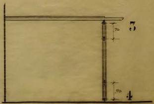
ΟΒΙΣ ΚΑ. 1/50
