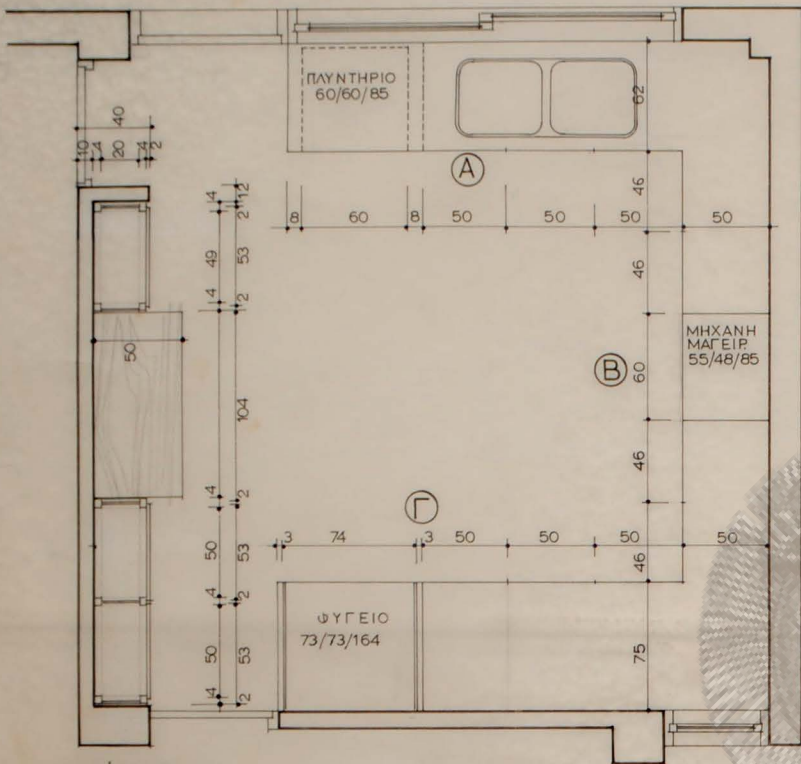
κάτοψις
