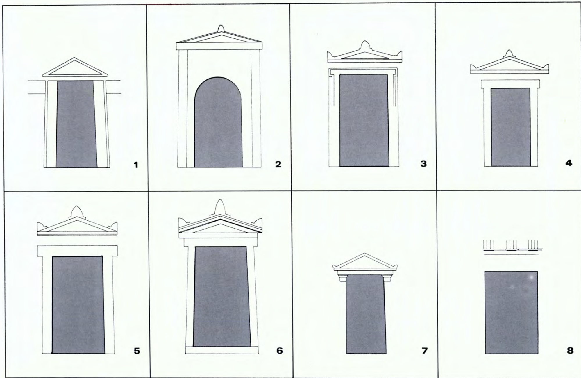
Σχέδ. 12. Προσόψεις λαξευτῶν θαλαμωτῶν τάφων Βεροίας: 1. Τάφος I οἰκοπέδου Ἐλευθεριάδη (κατ. ἀριθ. 2), 2. Τάφος οἰκοπέδου Βούλγαρη - Δούμου (κατ. ἀριθ. 4), 3. Τάφος οἰκοπέδου Σανοπούλου - Θεοδαρίδη (κατ. ἀριθ. 22), 4. Τάφος I οἰκοπέδου Μαυρίδη (κατ. ἀριθ. 18), 5. Τάφος οἰκοπέδου Χατζημάμογλου - Κοσμίδη (κατ. ἀριθ. 3), 6. Τάφος Συνοικισμοῦ Καλλιθέας (κατ. ἀριθ. 20), 7. Τάφος I οἰκοπέδου Γυμνασίου Ἀρρένων (κατ. ἀριθ. 23), 8. Τάφος II οἰκοπέδου Πισσᾶ (κατ. ἀριθ. 15).
