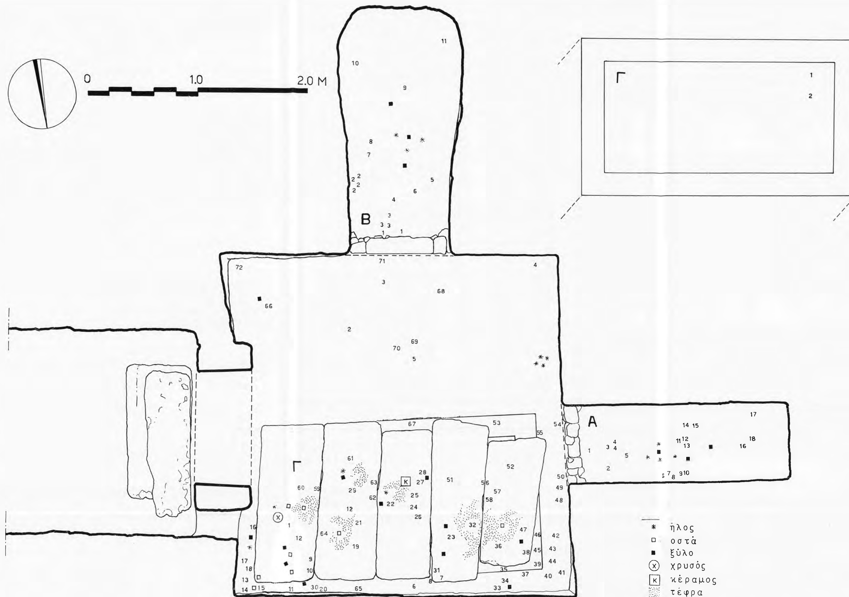
Σχέδ. IV. Θαλαμῶτος τάφος οἰκοπέδου Θ. Σανοπούλου - Α. Θεοδορίδη. Κάτοψη μέ τή θέση τῶν κτερισμάτων.
