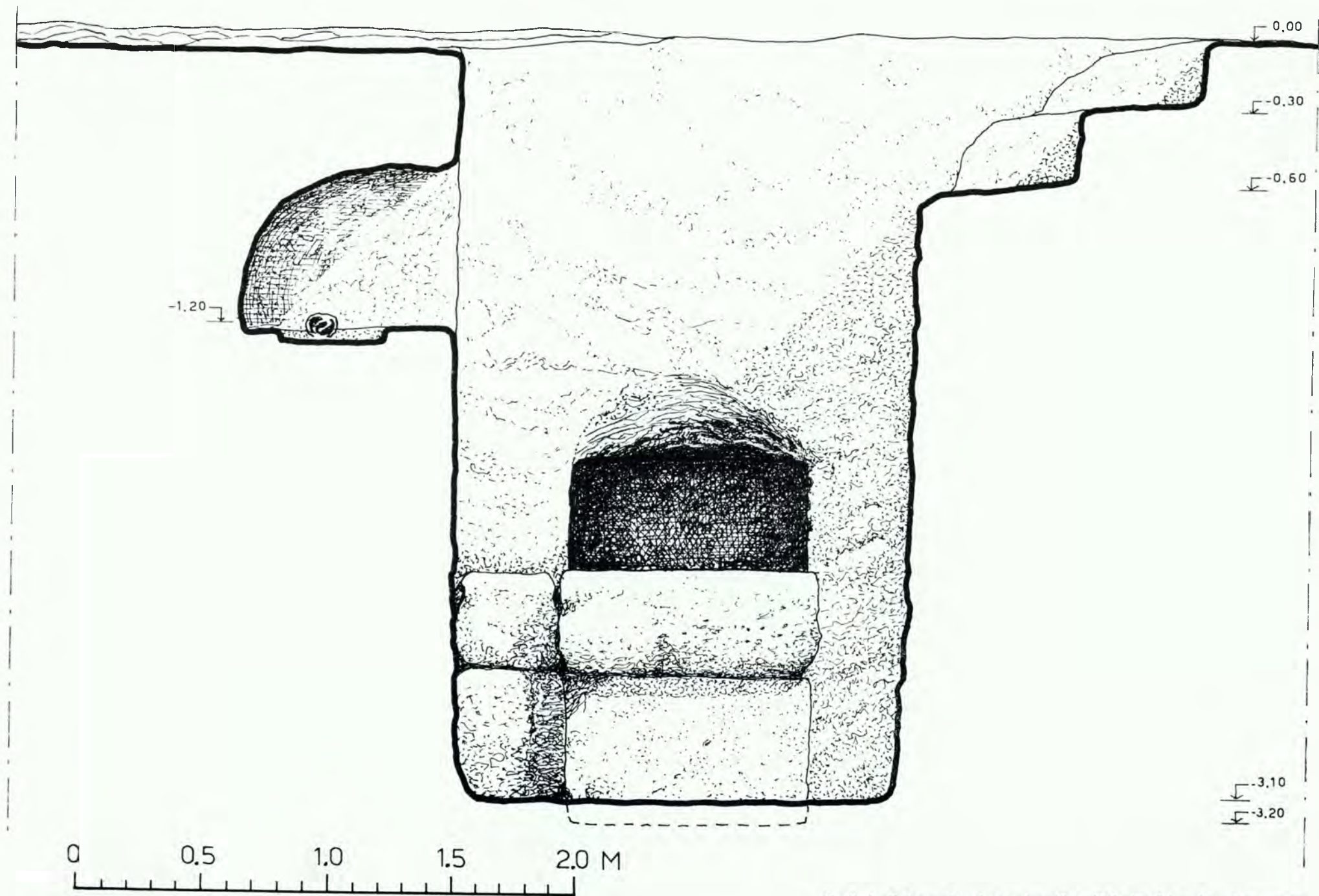
Σχέδ. 5. Θαλαμωτός τάφος οικοπέδου αδελφών Θώμογλου. Τομή Β-Β'.
