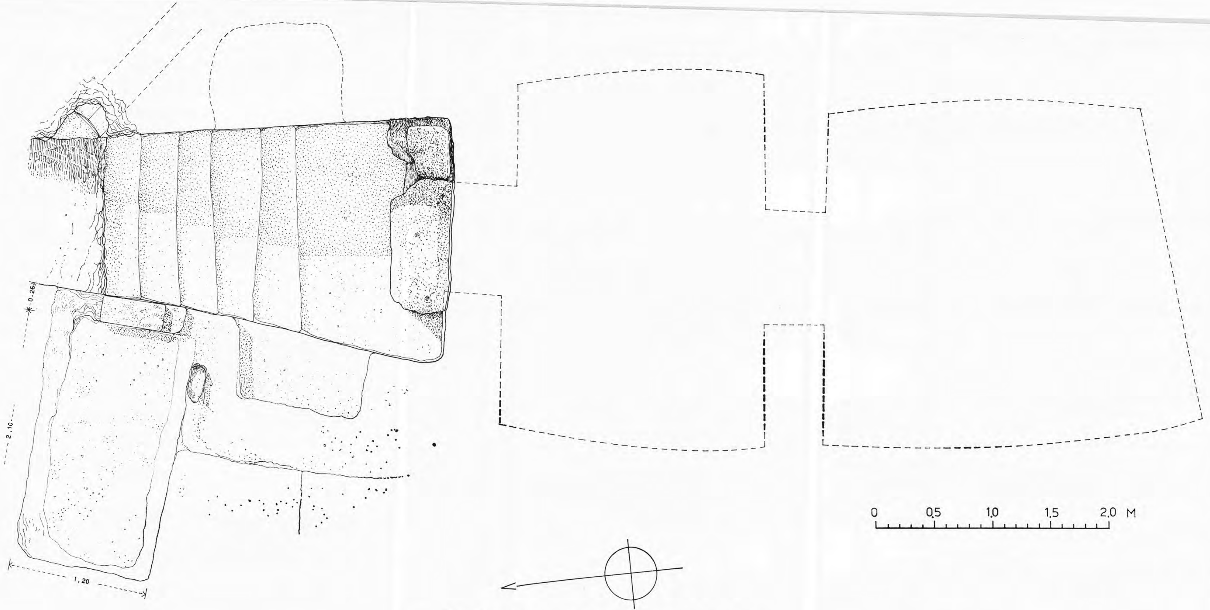
Σχέδ. VII. Θαλαμωτός τάφος οικοπέδου αδελφών Θάμογλου. Κάτοψη δρόμου και κλασικών τάφων.
