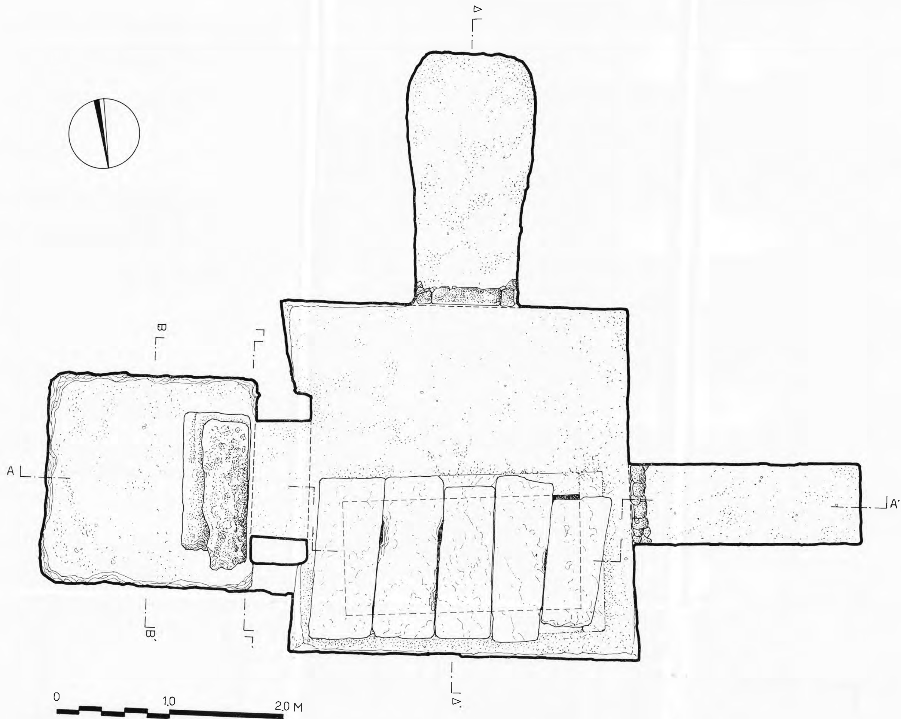
Σχέδ. II. Θαλαμωτός τάφος οικοπέδου Θ. Σανοπούλου -'Α. Θεοδωρίδη. Κάτοψη.
