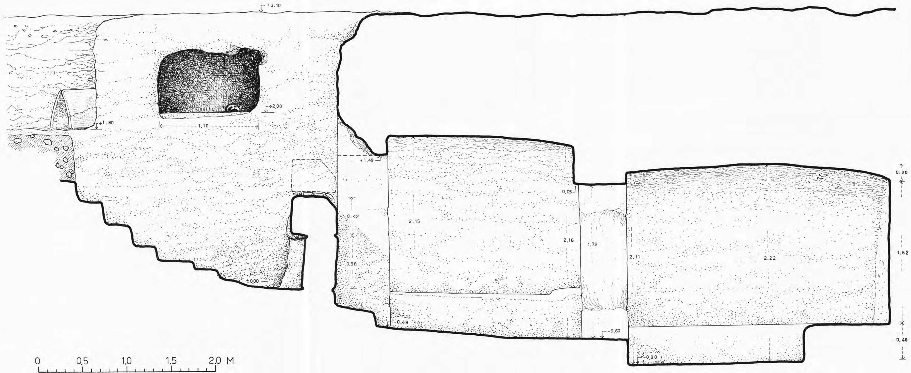
Σχέδ. VIII. Θαλαματός τάφος οικόπεδου αδελφών Θώμογλου. Τομή Α-Α'.
