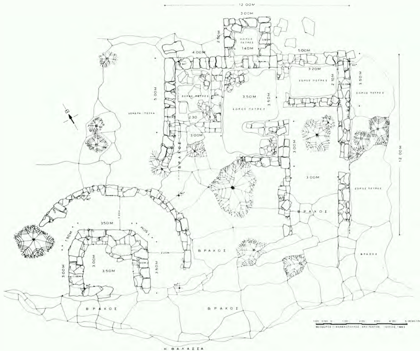
Σχέδ. 112. Φυλακεία Ξεροπήγαδου. Κάτοψη.
