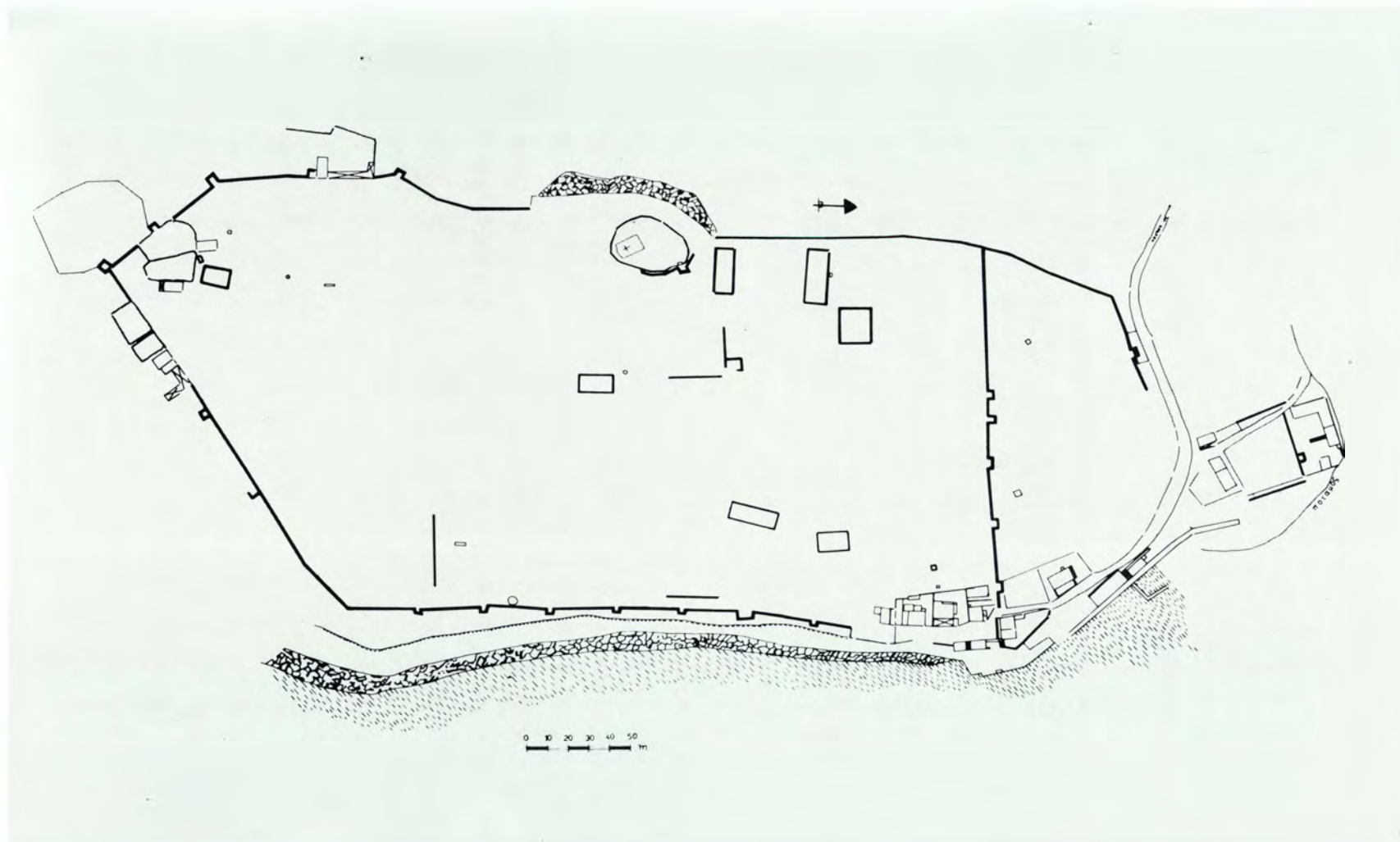
Σχέδ. 12. Νησί Αγίου Ανδρέα. Η οχύρωση του οικισμού (σχέδ. Β. Ξαφίτσα).
